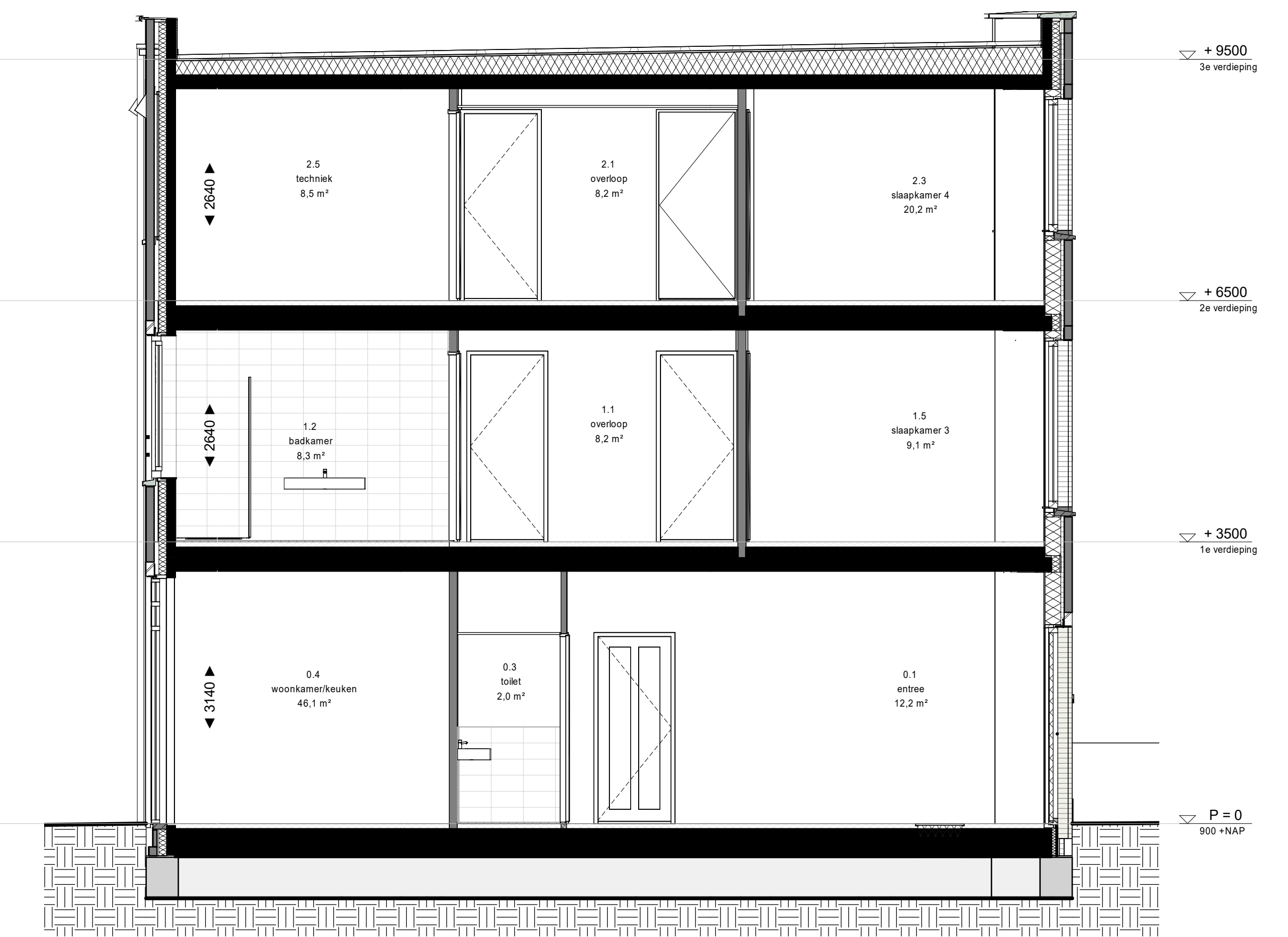
doorsnede
