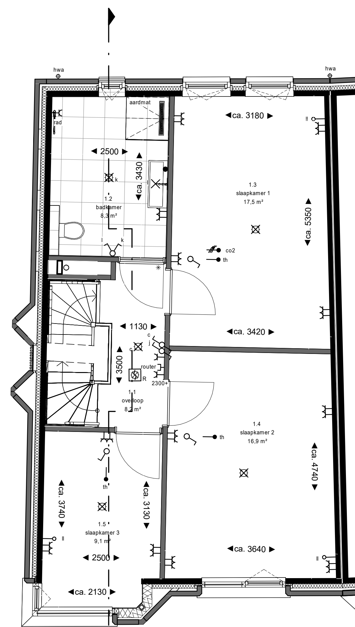
1e verdieping
