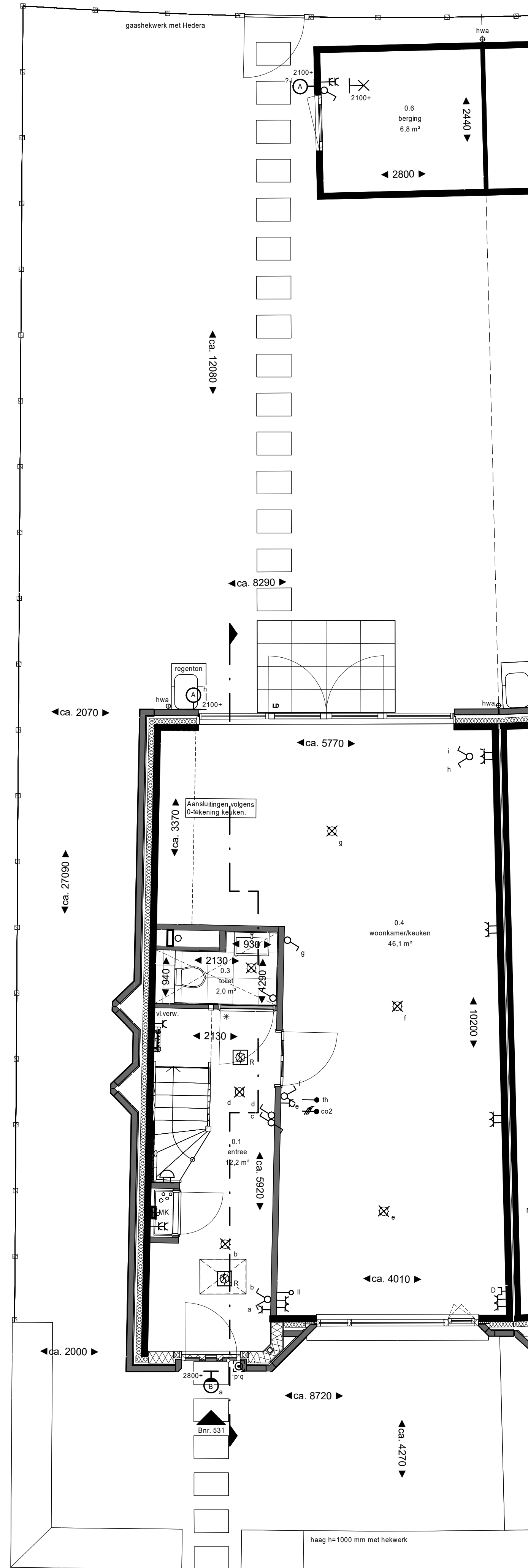
begane grond
