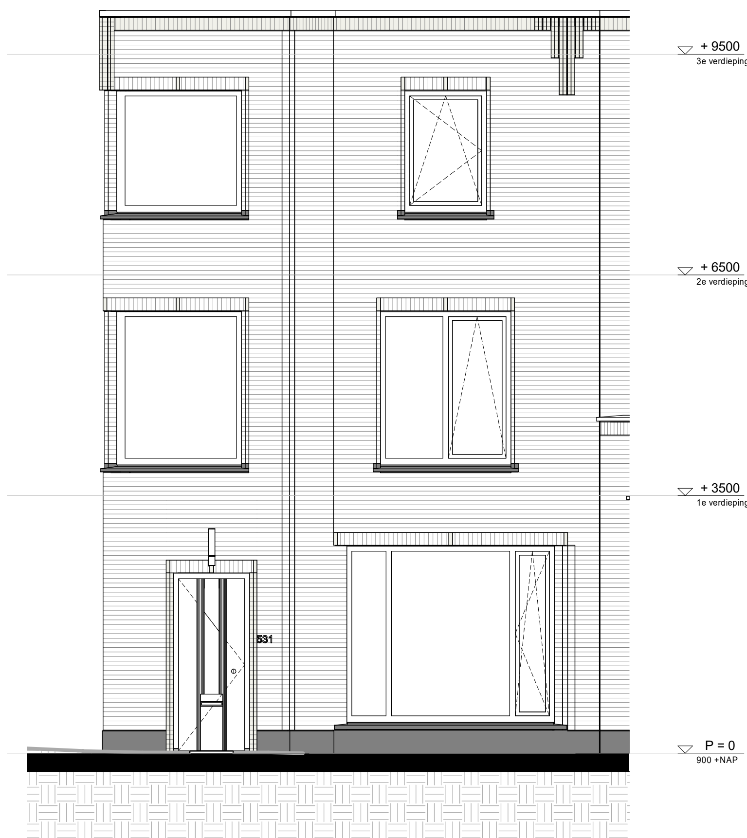
voorgevel
