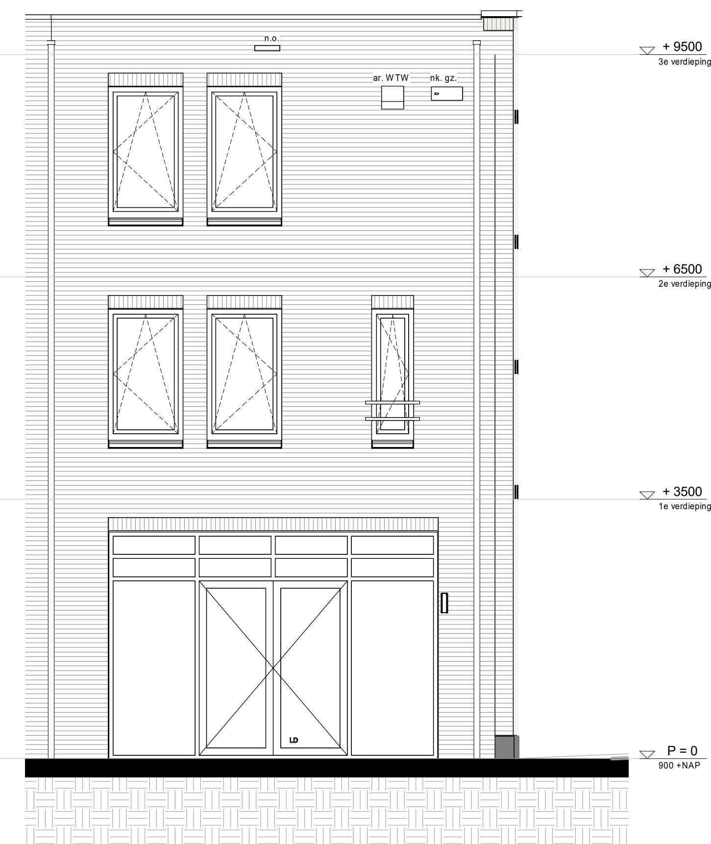
achtergevel
