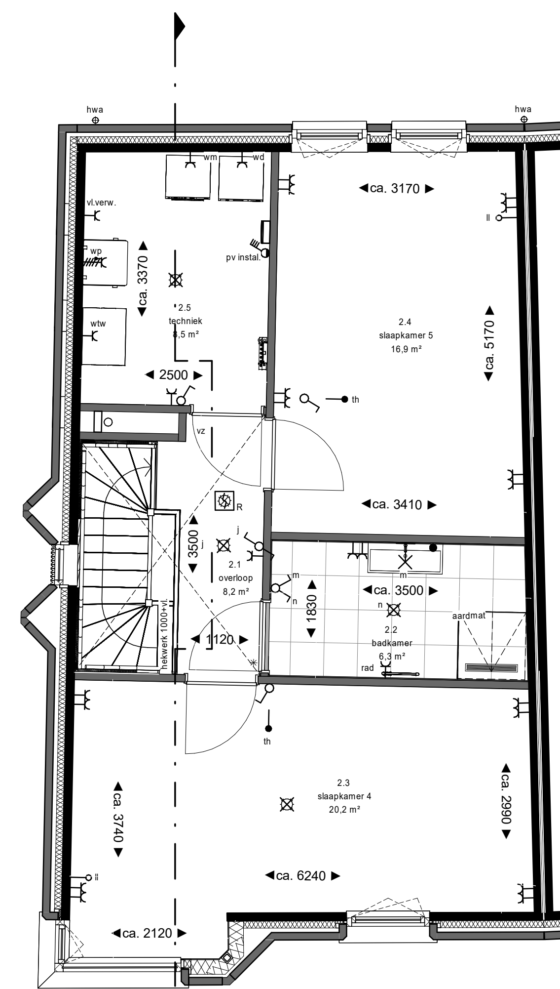
2e verdieping
