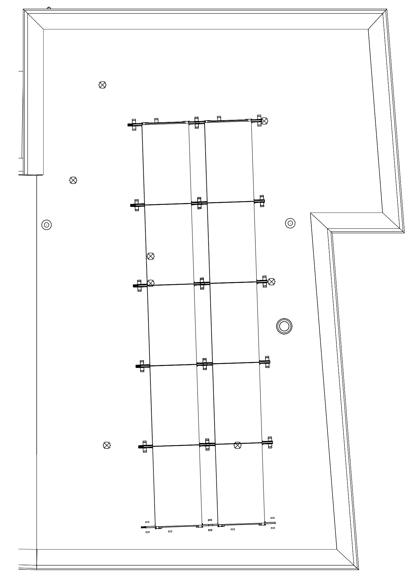
dakaanzicht
