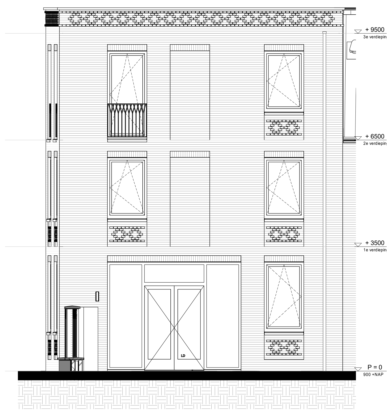
achtergevel
