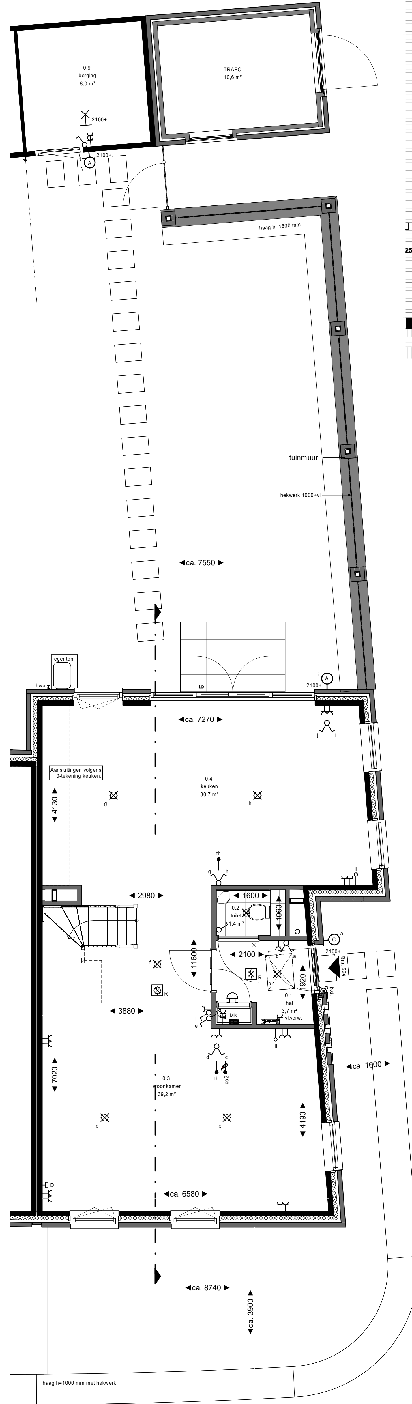
begane grond
