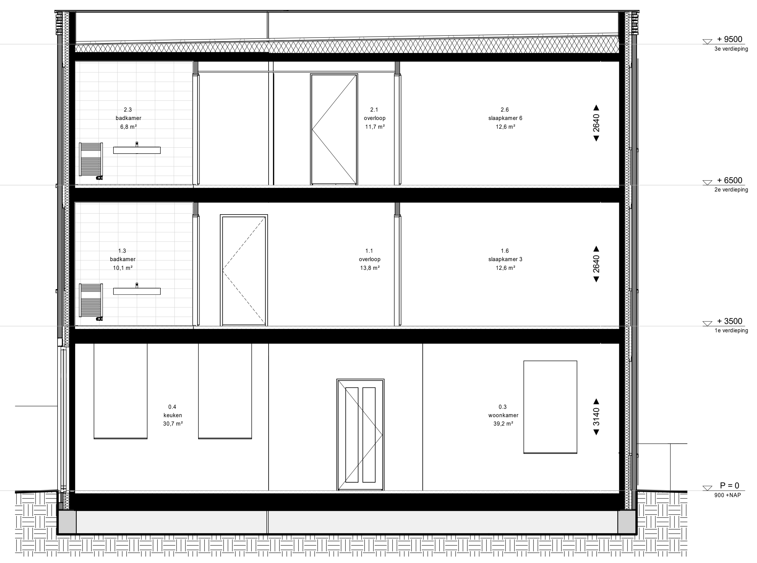
doorsnede
