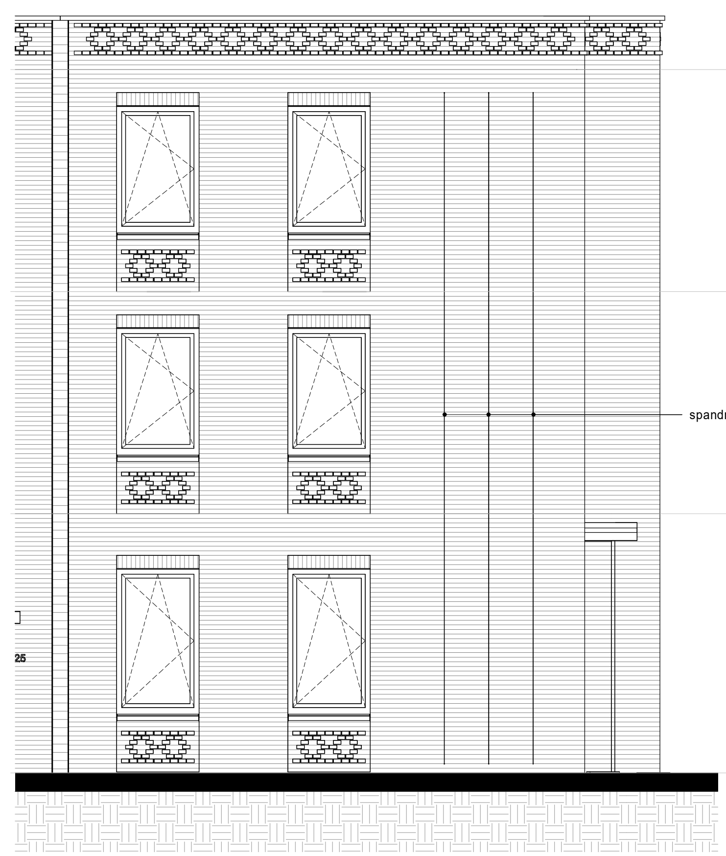
voorgevel
