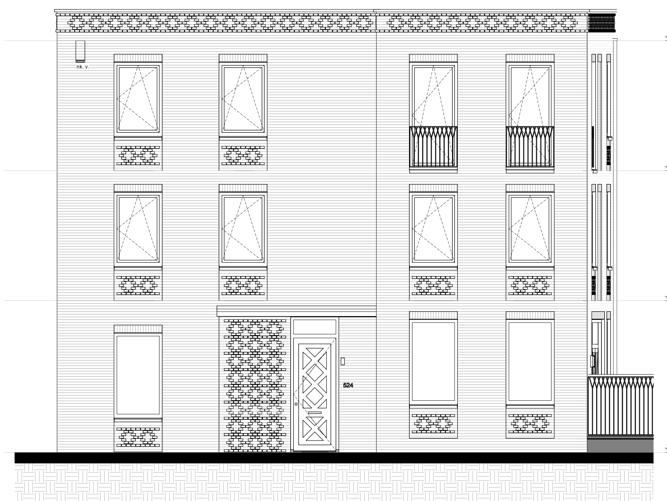
zijgevel
