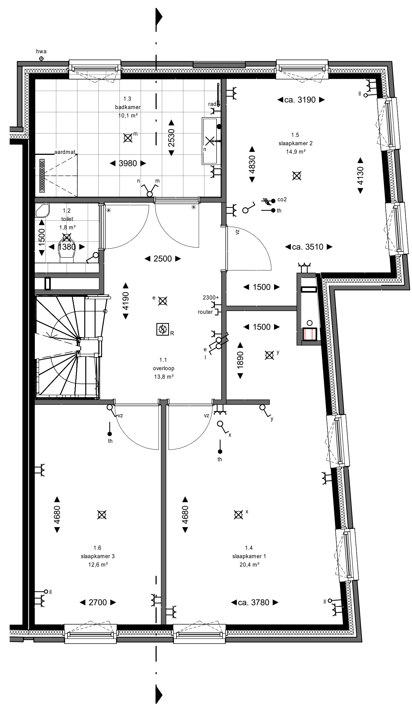
1e verdieping
