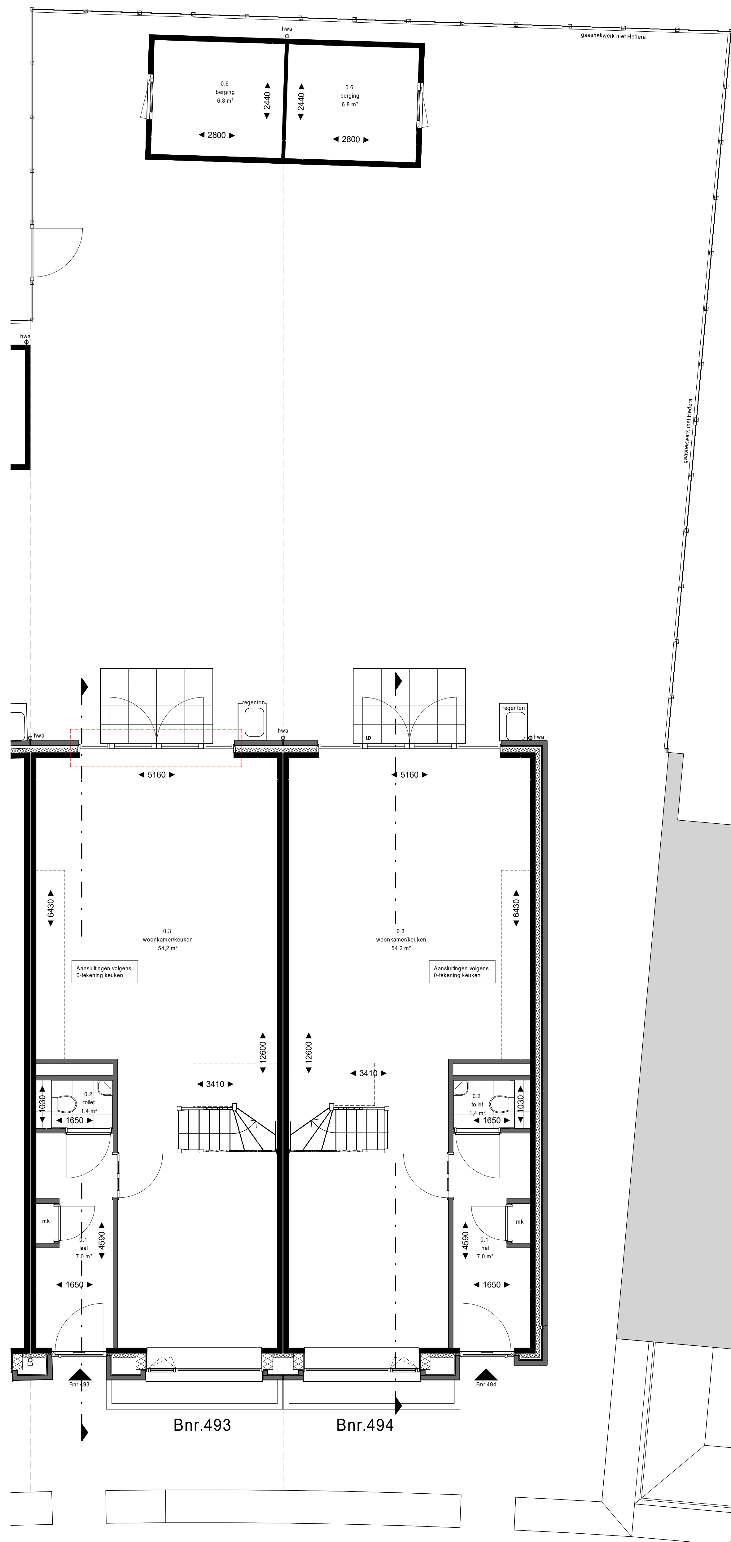
begane grond - Optie uitbouw begane grond 2.40 m 2
