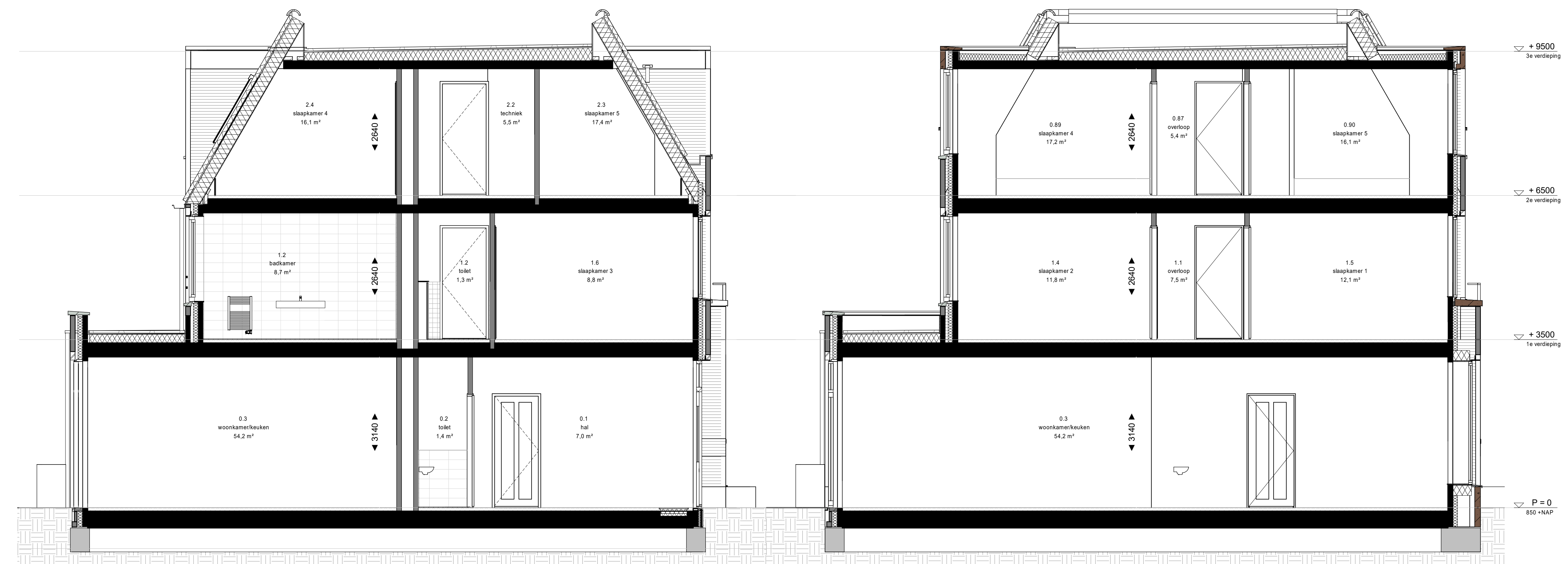
doorsnede Bnr.493 - Optie uitbouw begane grond 2.40 m 2
