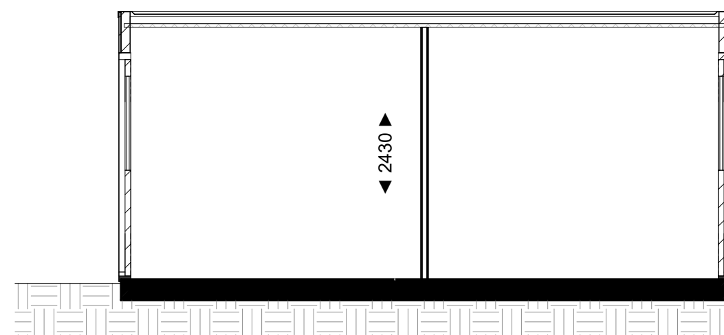
doorsnede
