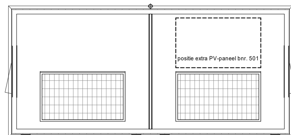
dakaanzicht
