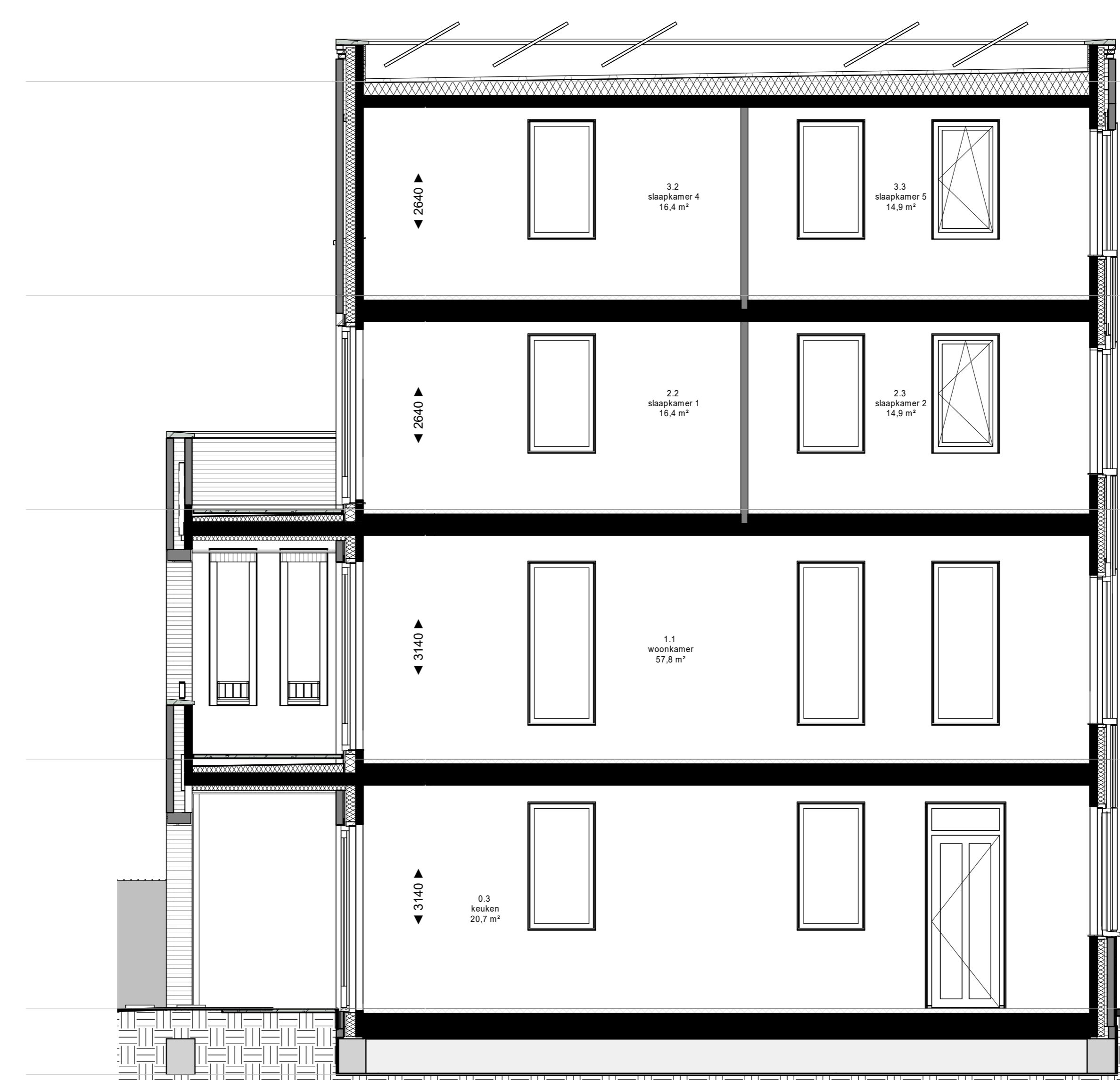
doorsnede
