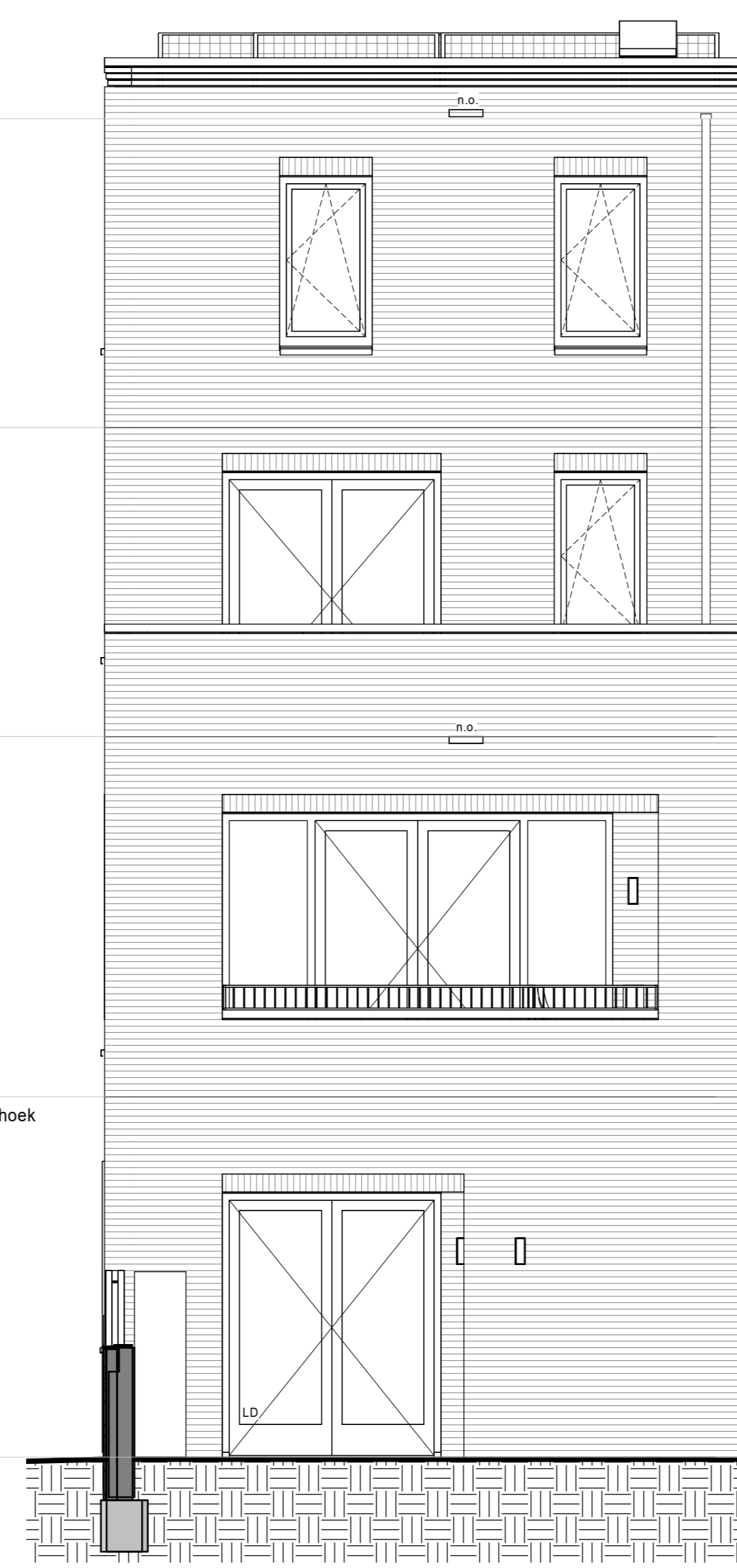
achtergevel
