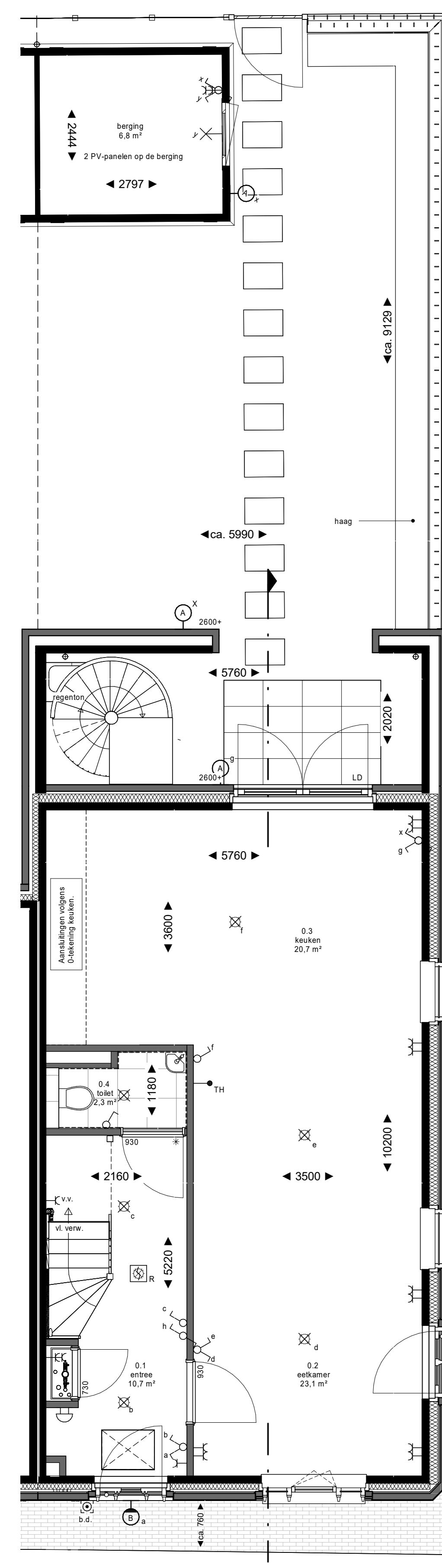
begane grond
