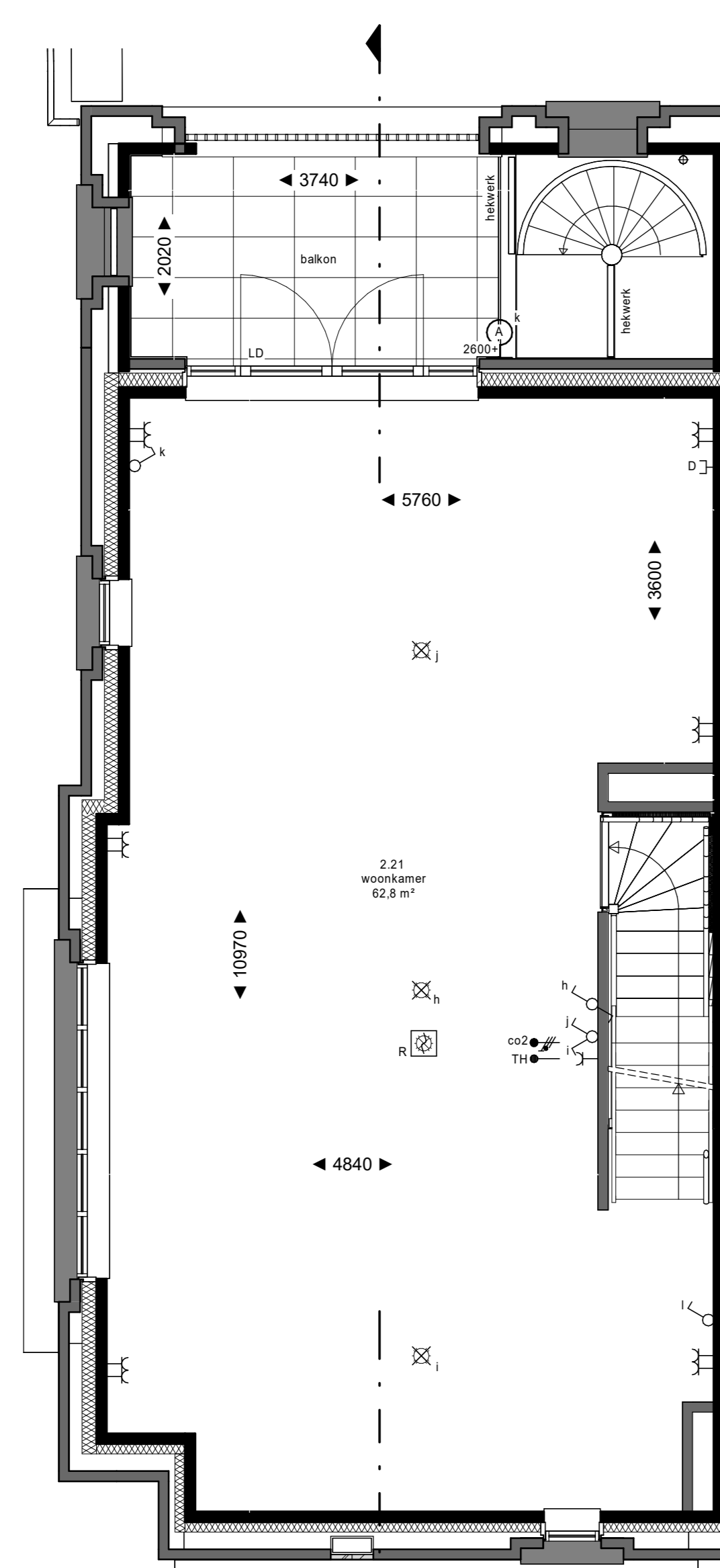
1e verdieping
