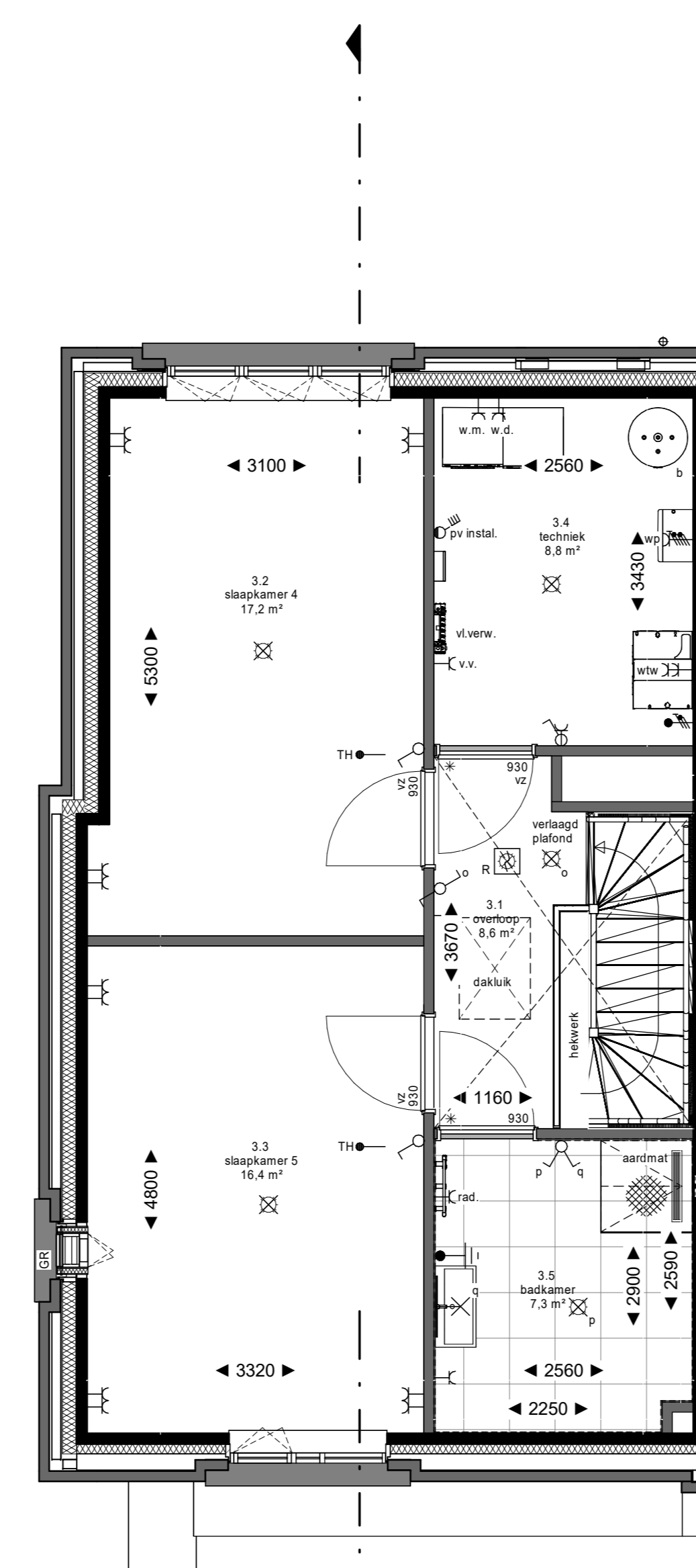
3e verdieping
