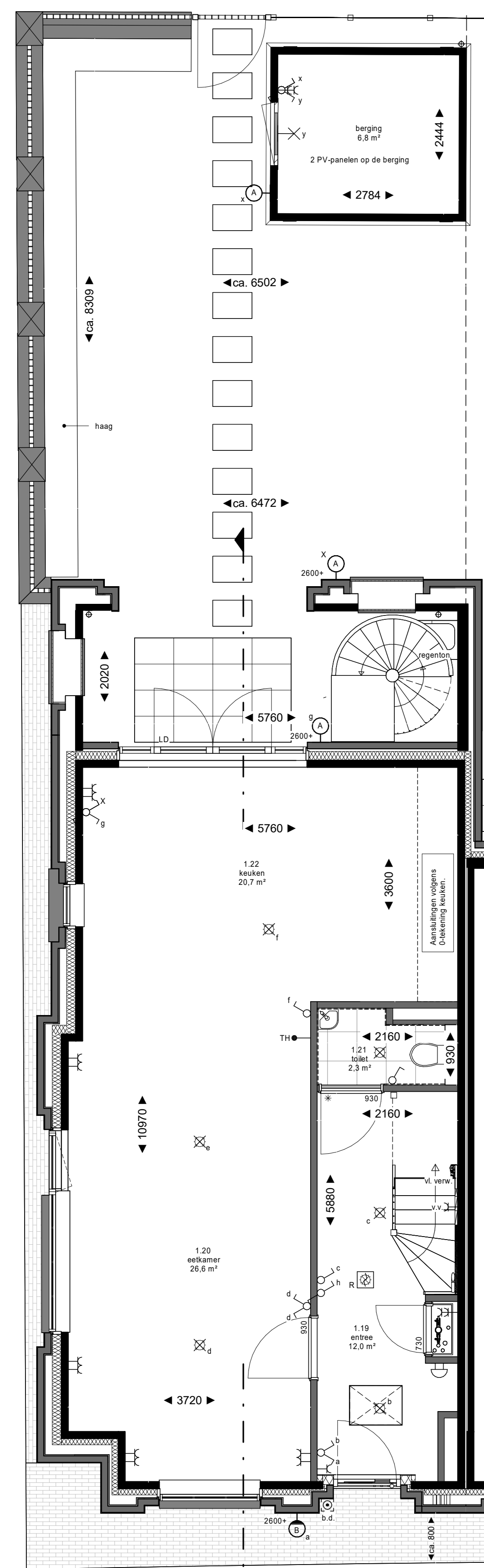
begane grond
