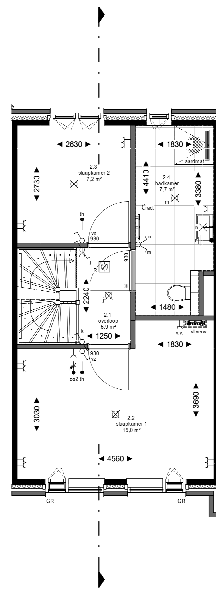
2e verdieping
