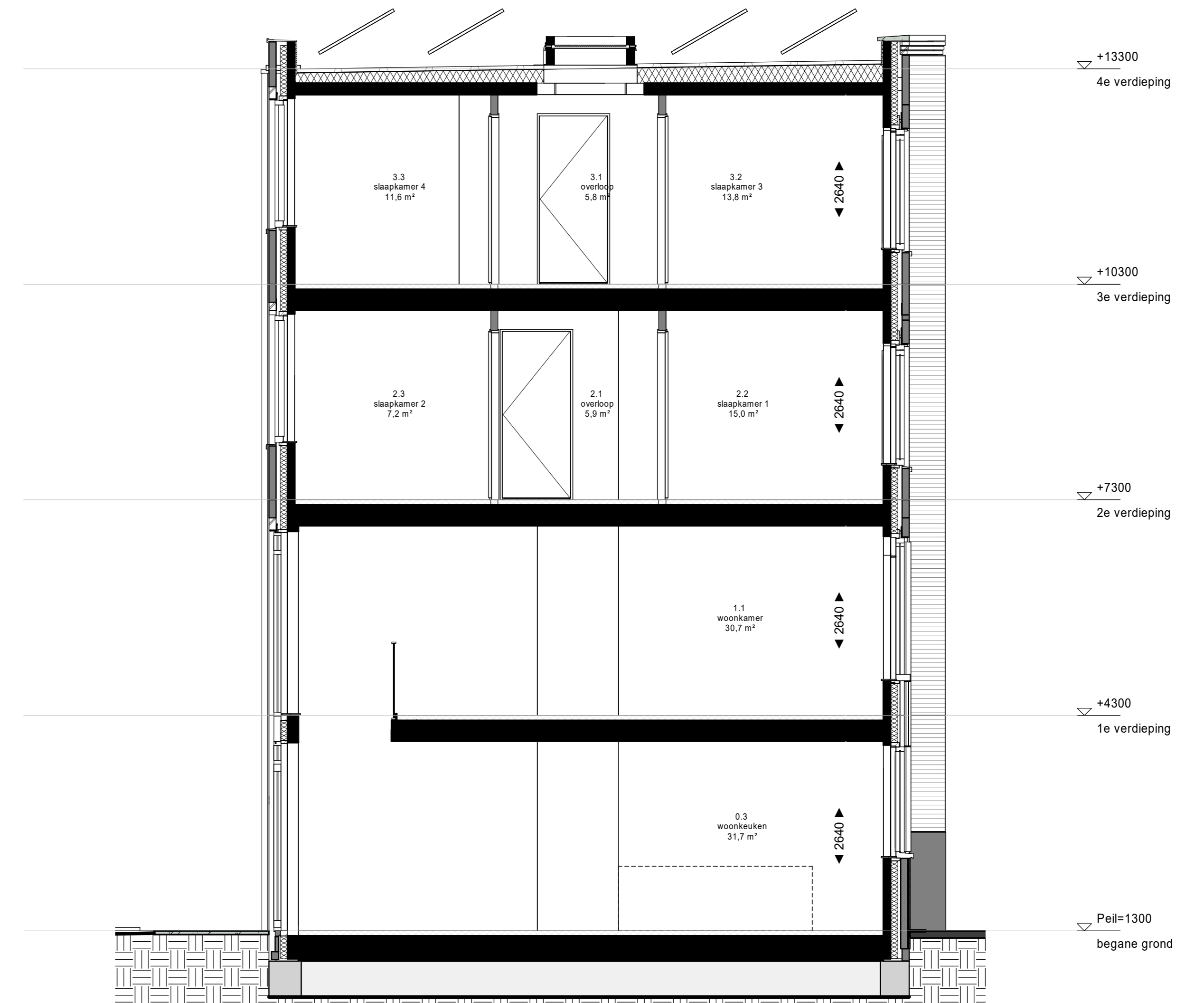
doorsnede
