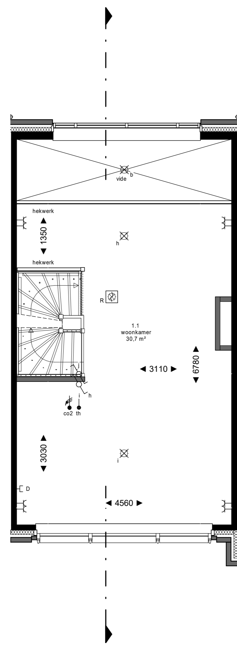
1e verdieping
