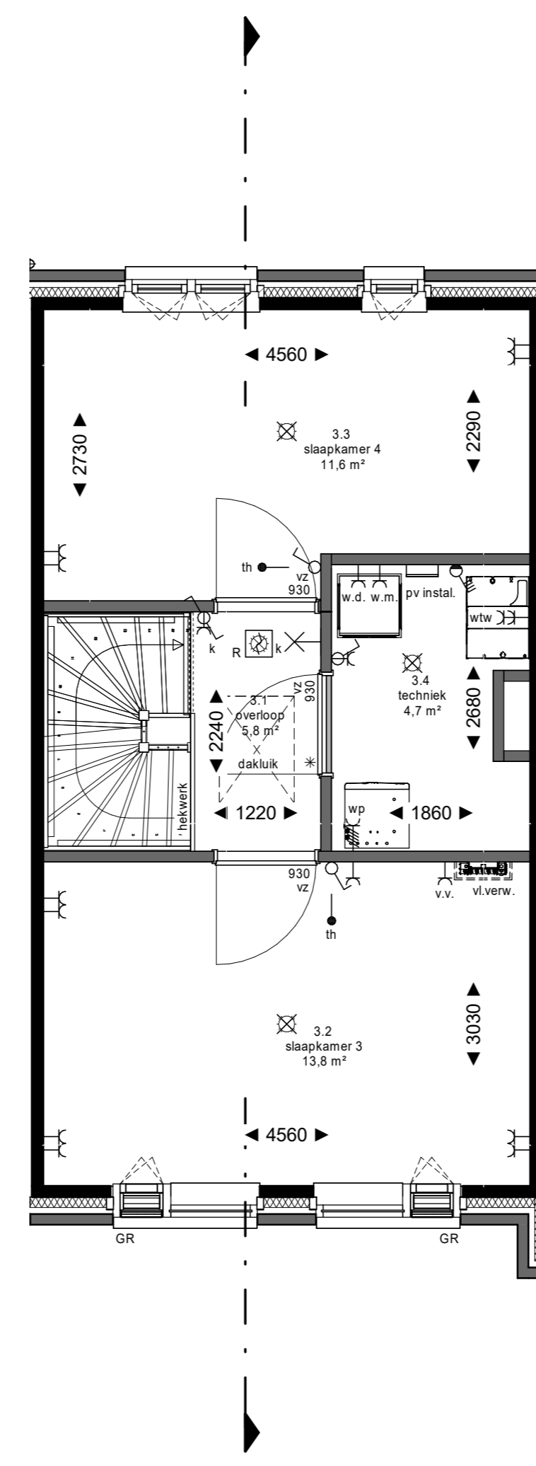
3e verdieping
