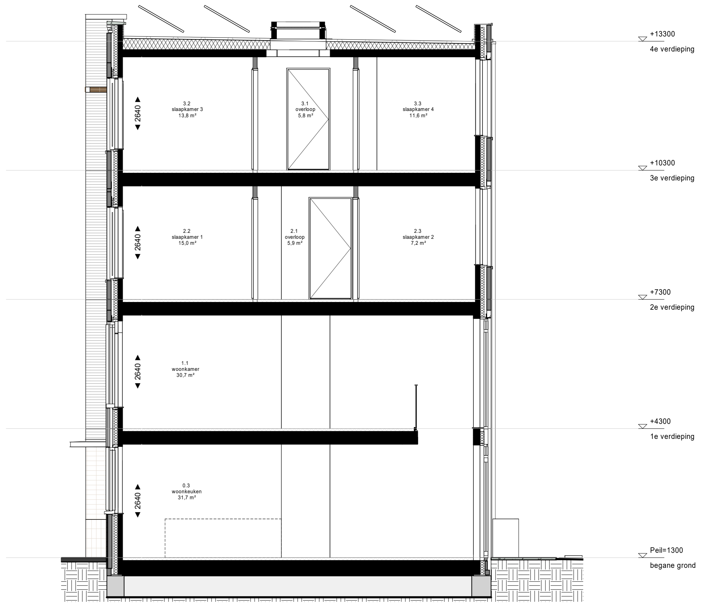
doorsnede
