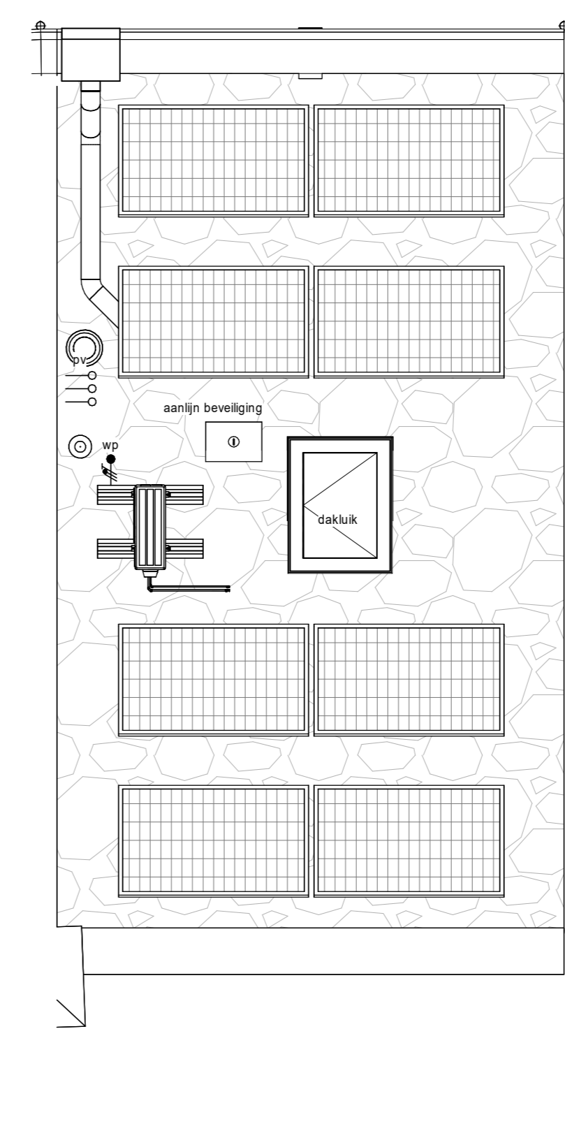
dakaanzicht
