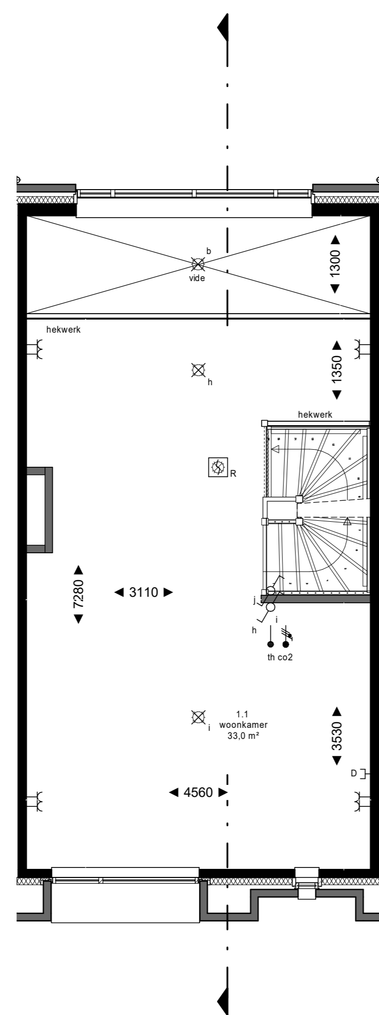
1e verdieping
