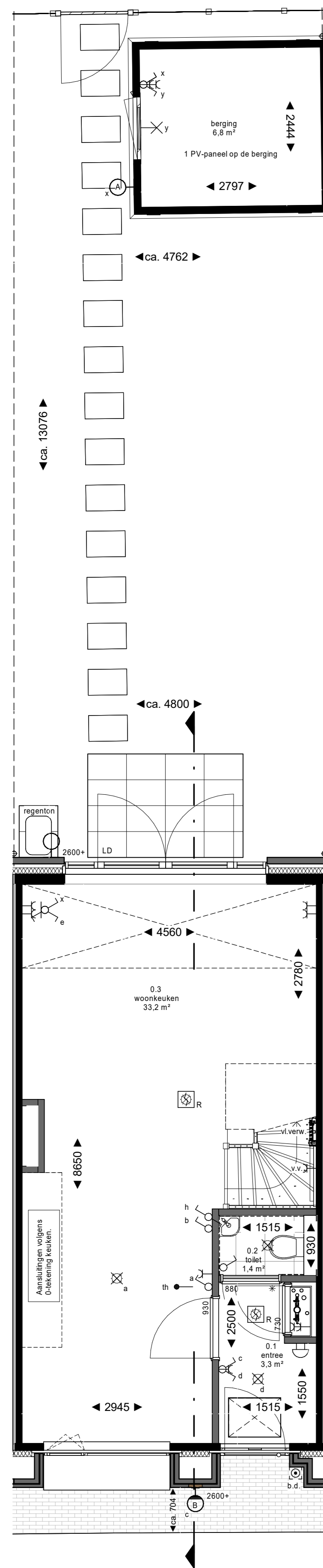
begane grond
