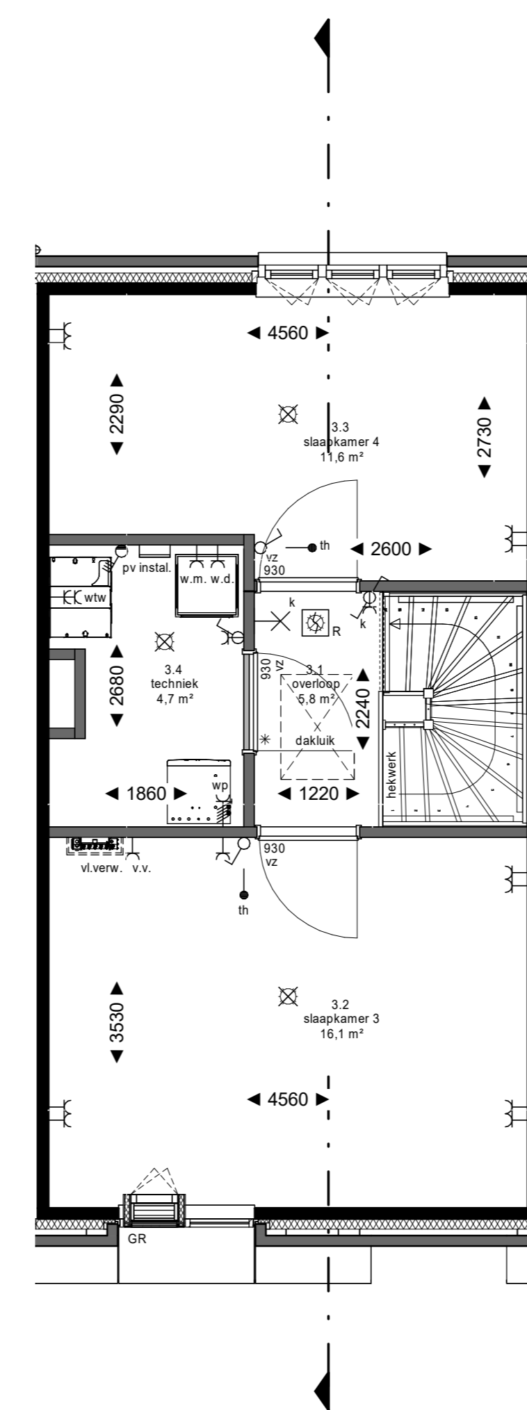
3e verdieping
