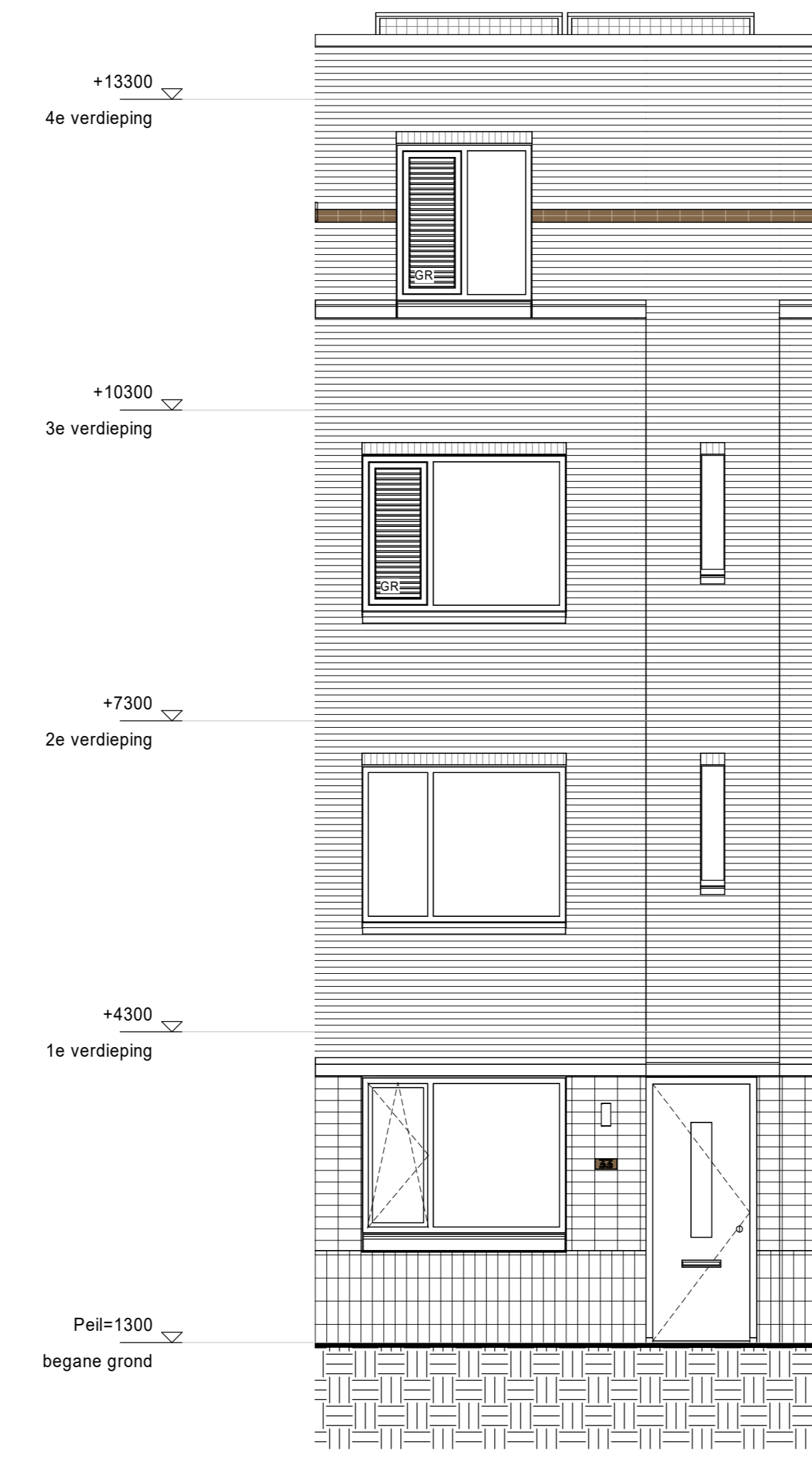
voorgevel
