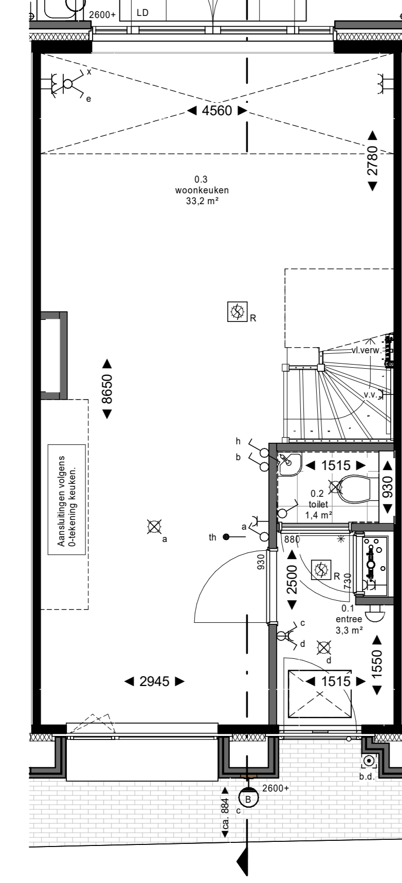
begane grond
