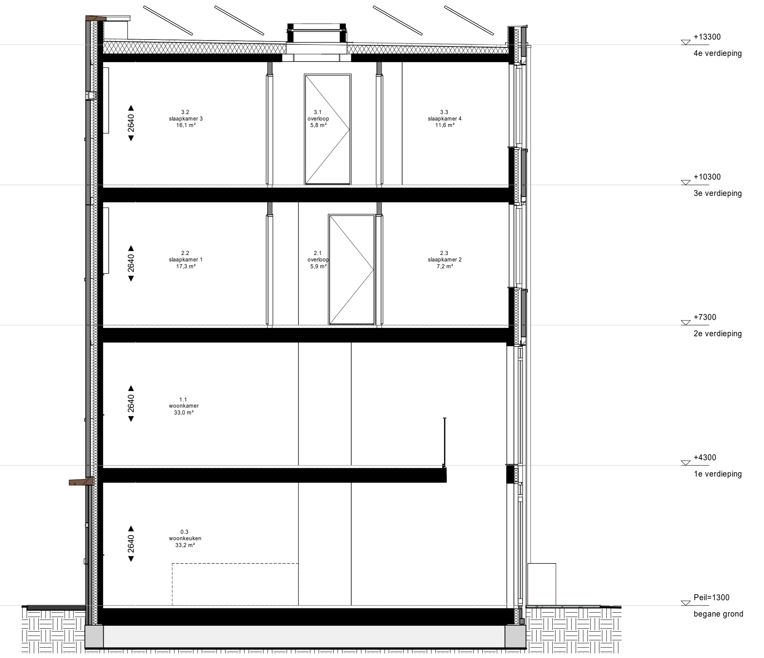
doorsnede
