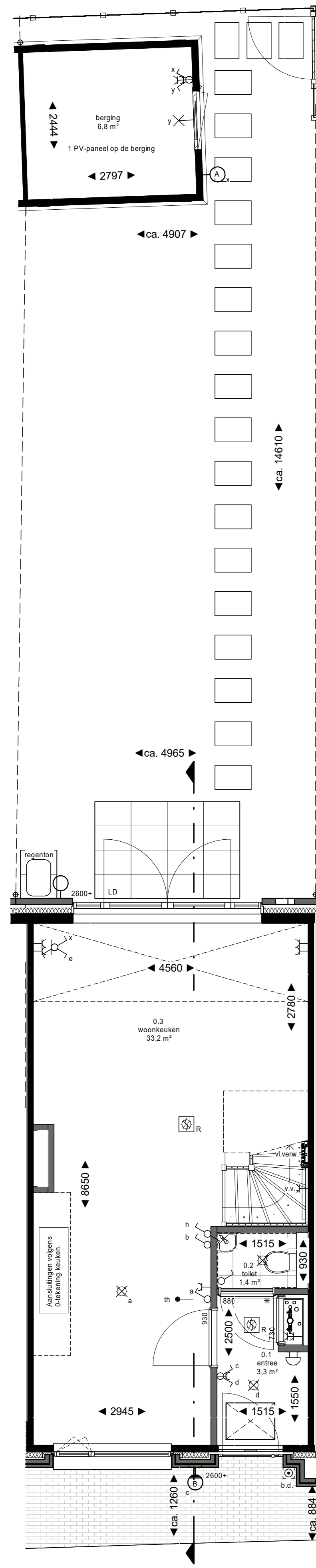
begane grond
