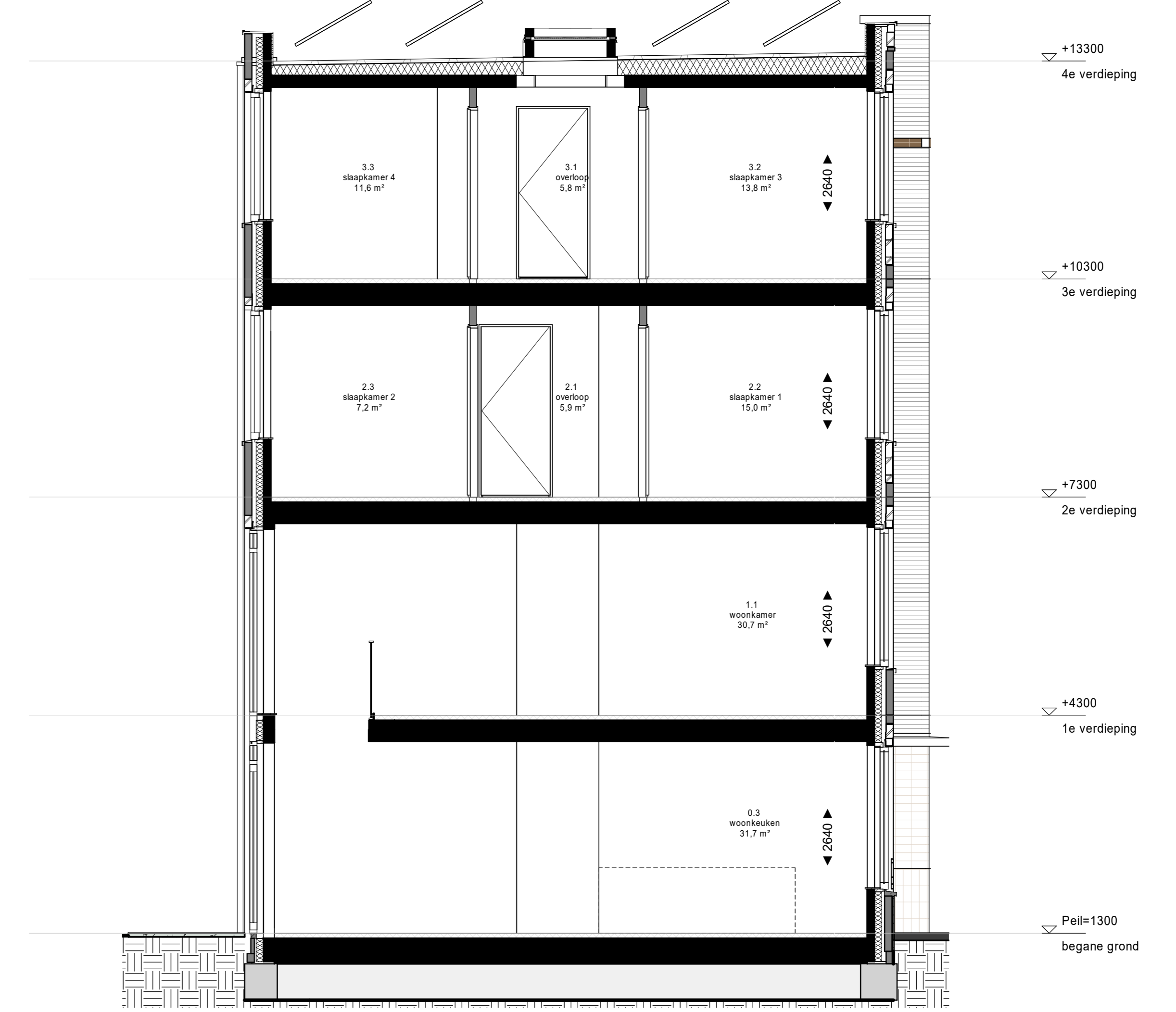
doorsnede
