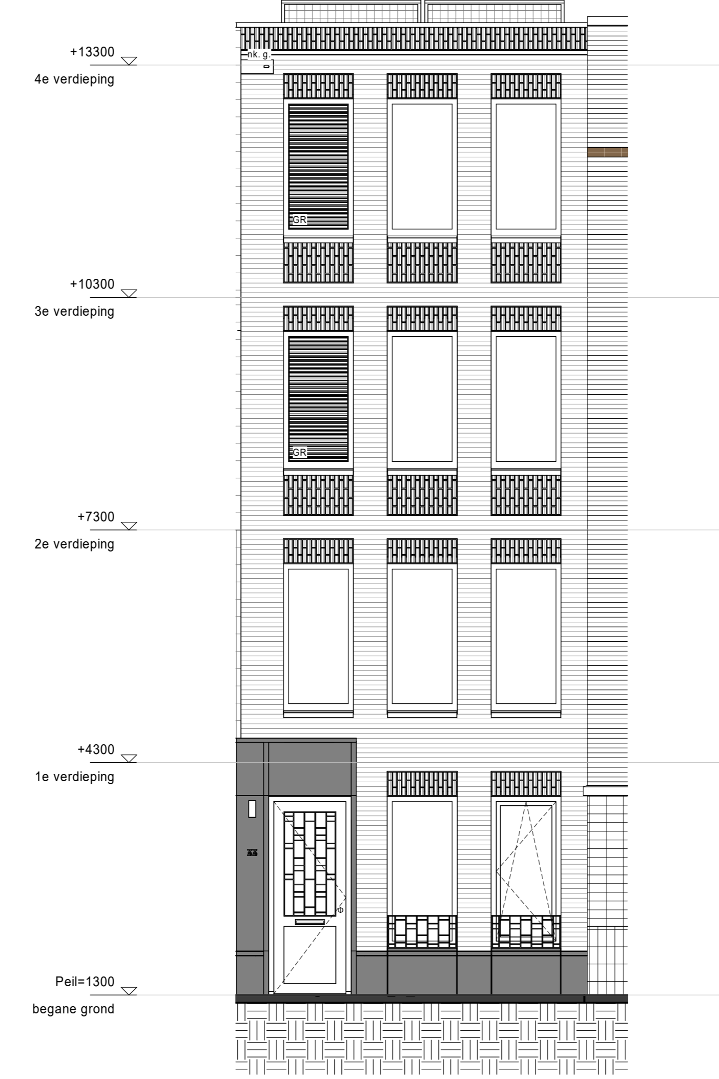
voorgevel
