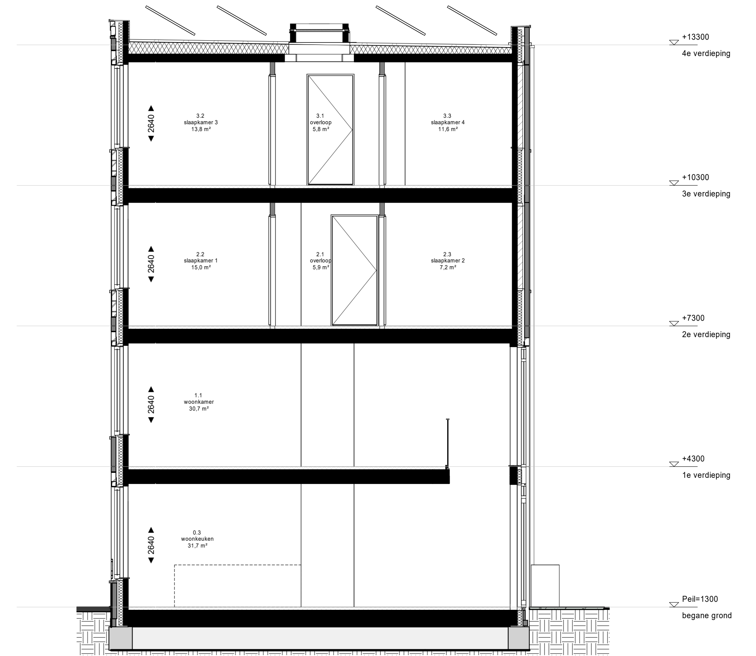
doorsnede
