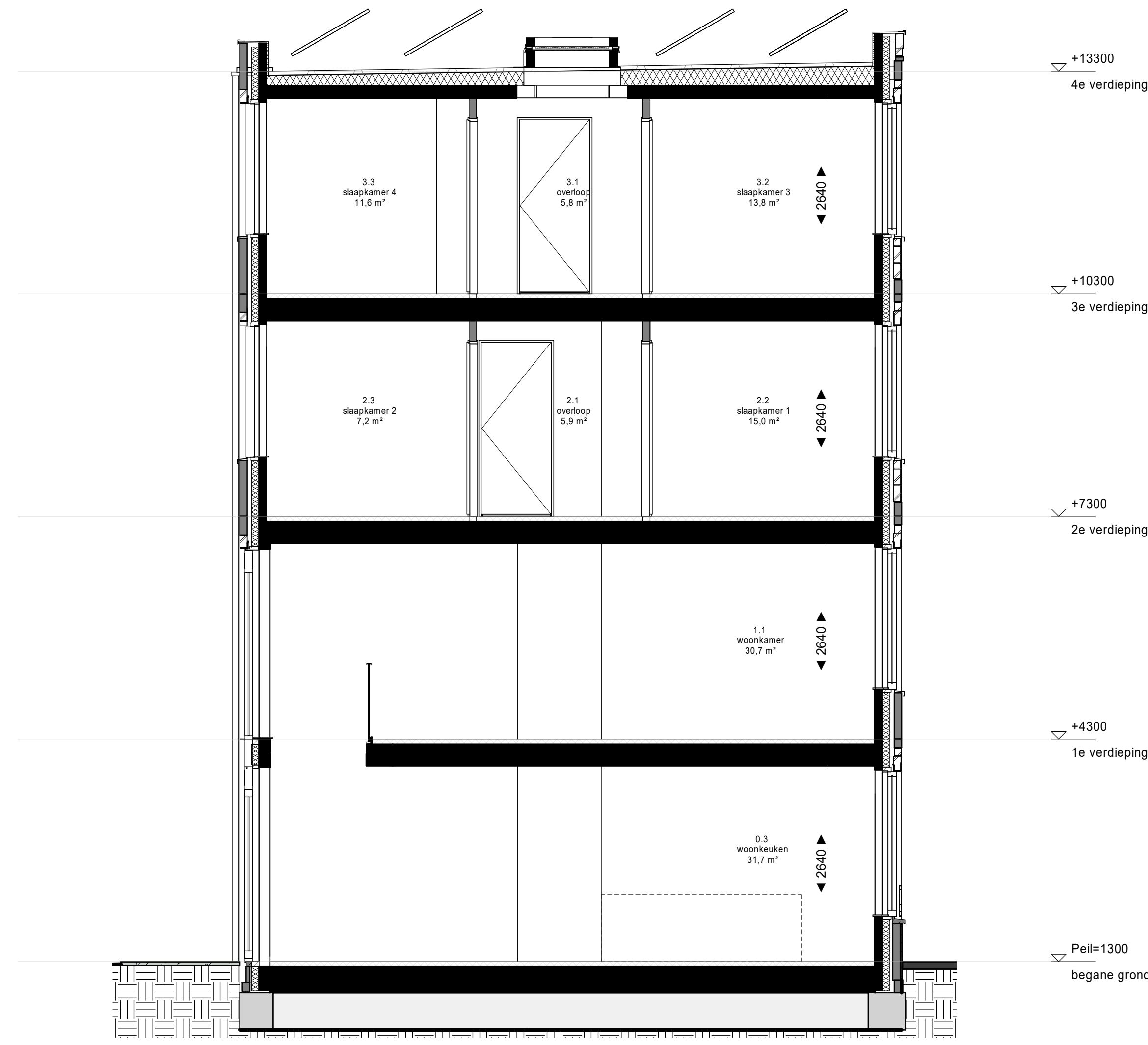
doorsnede
