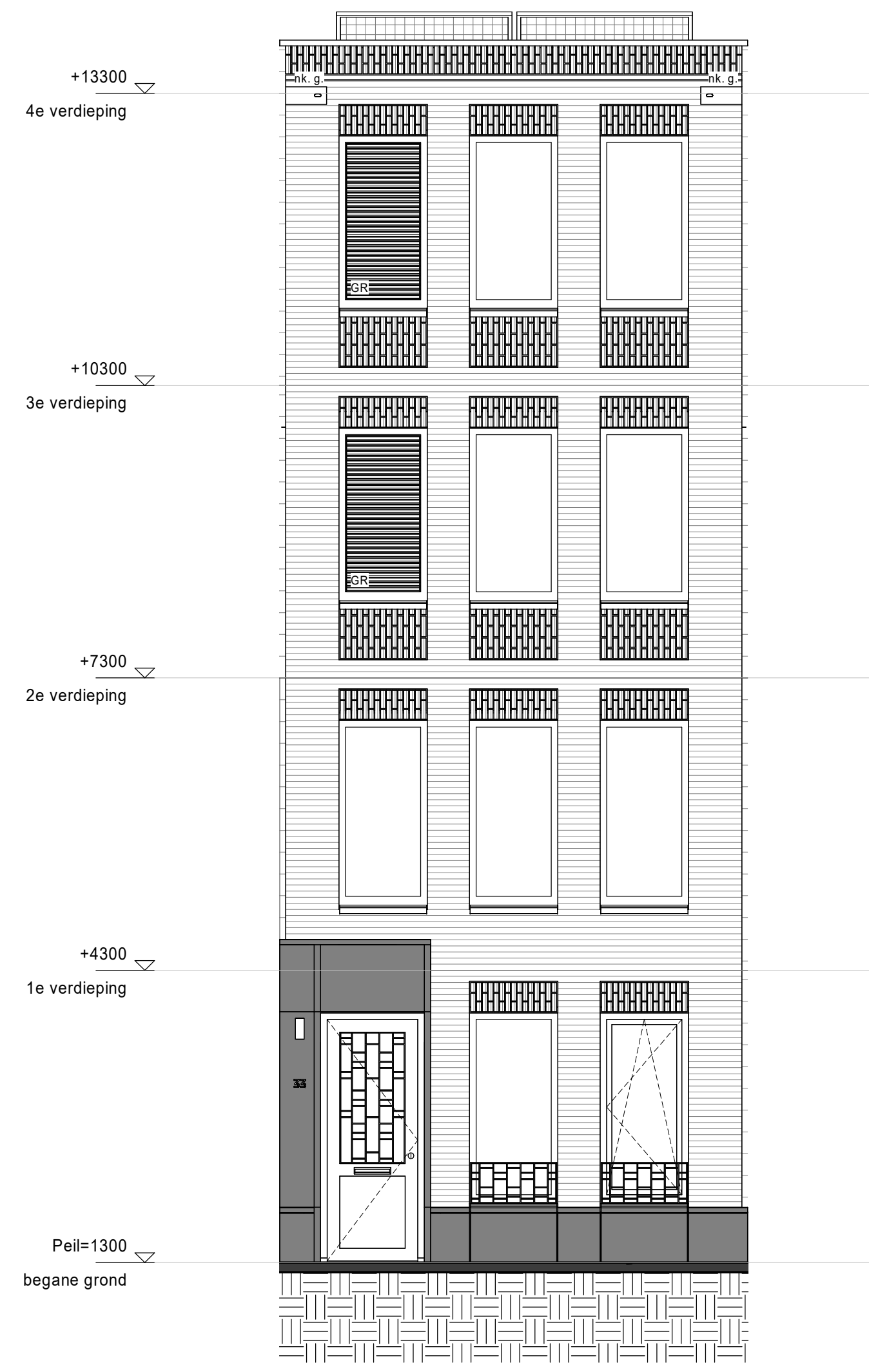
voorgevel
