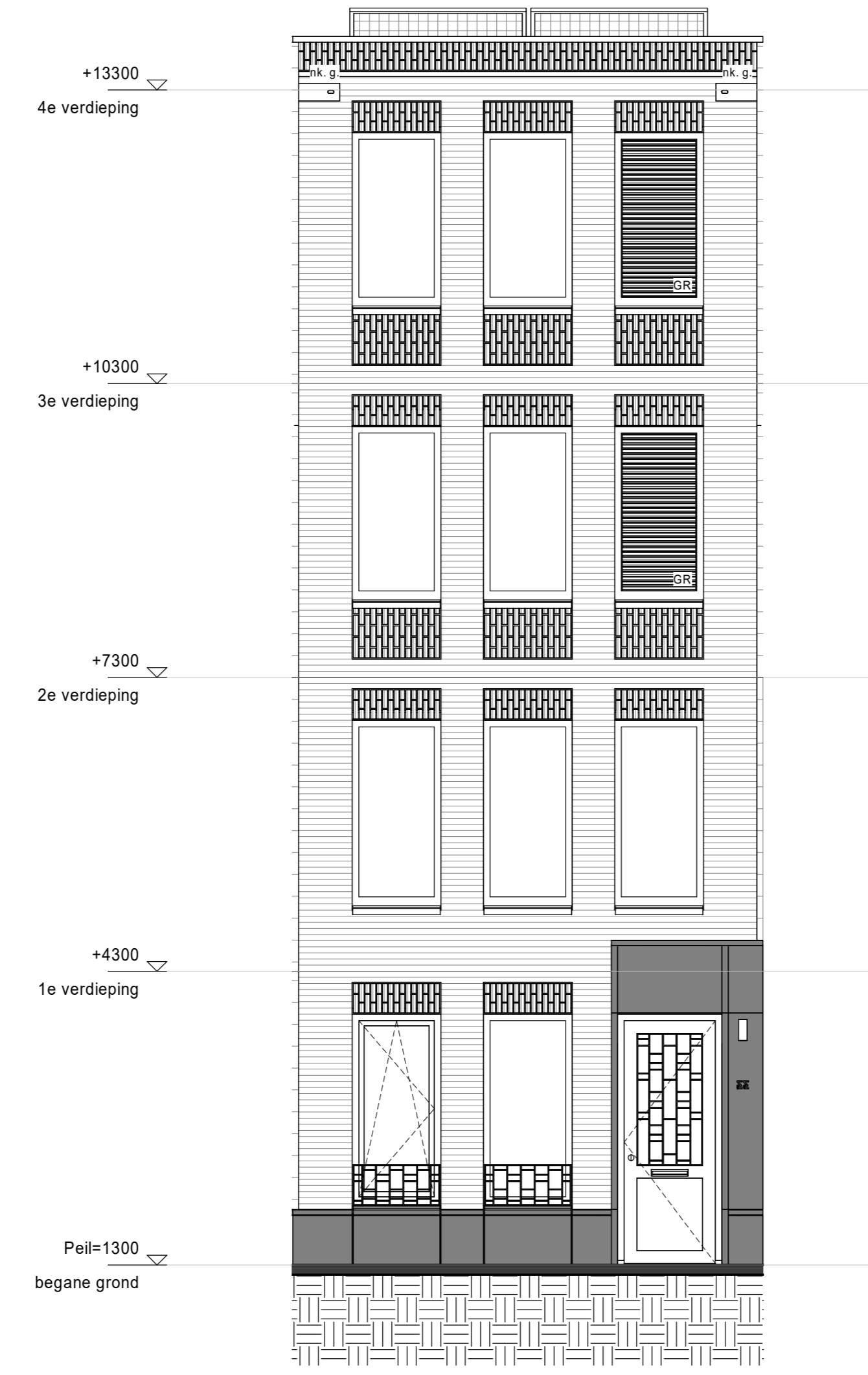
voorgevel
