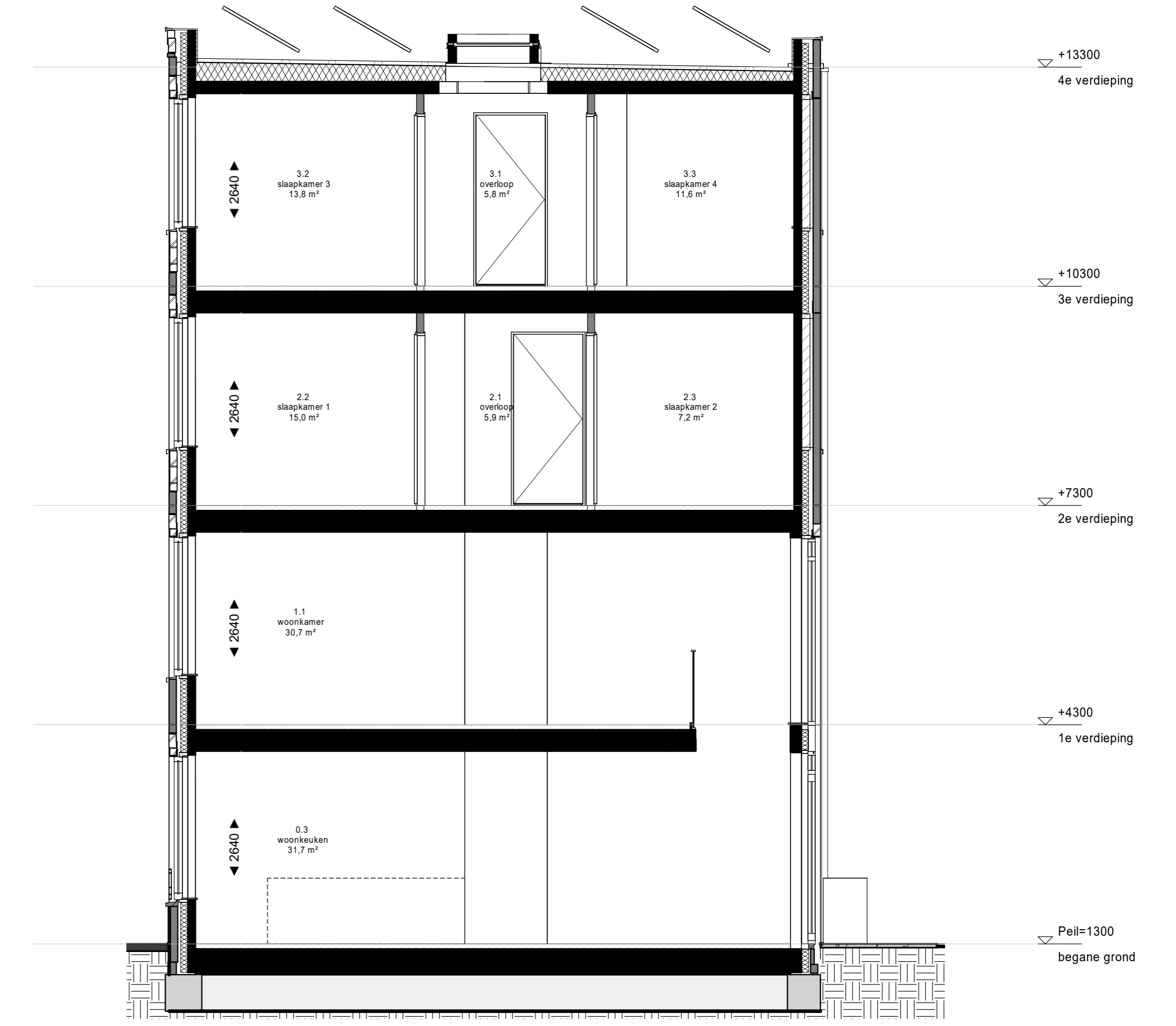
doorsnede
