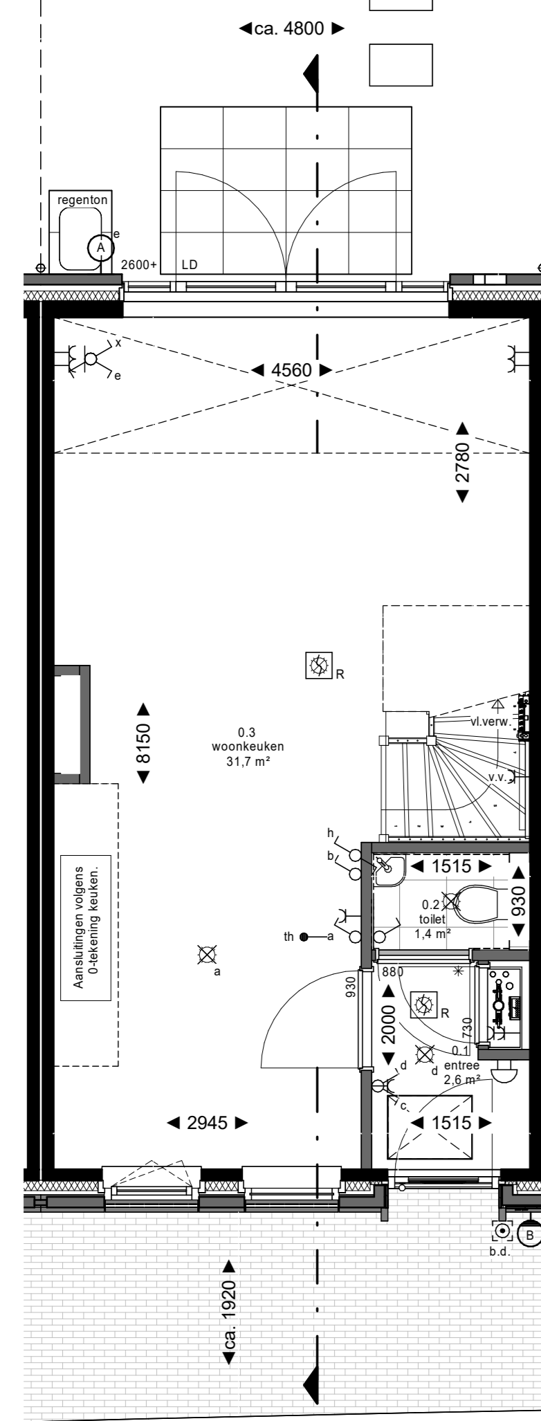
begane grond
