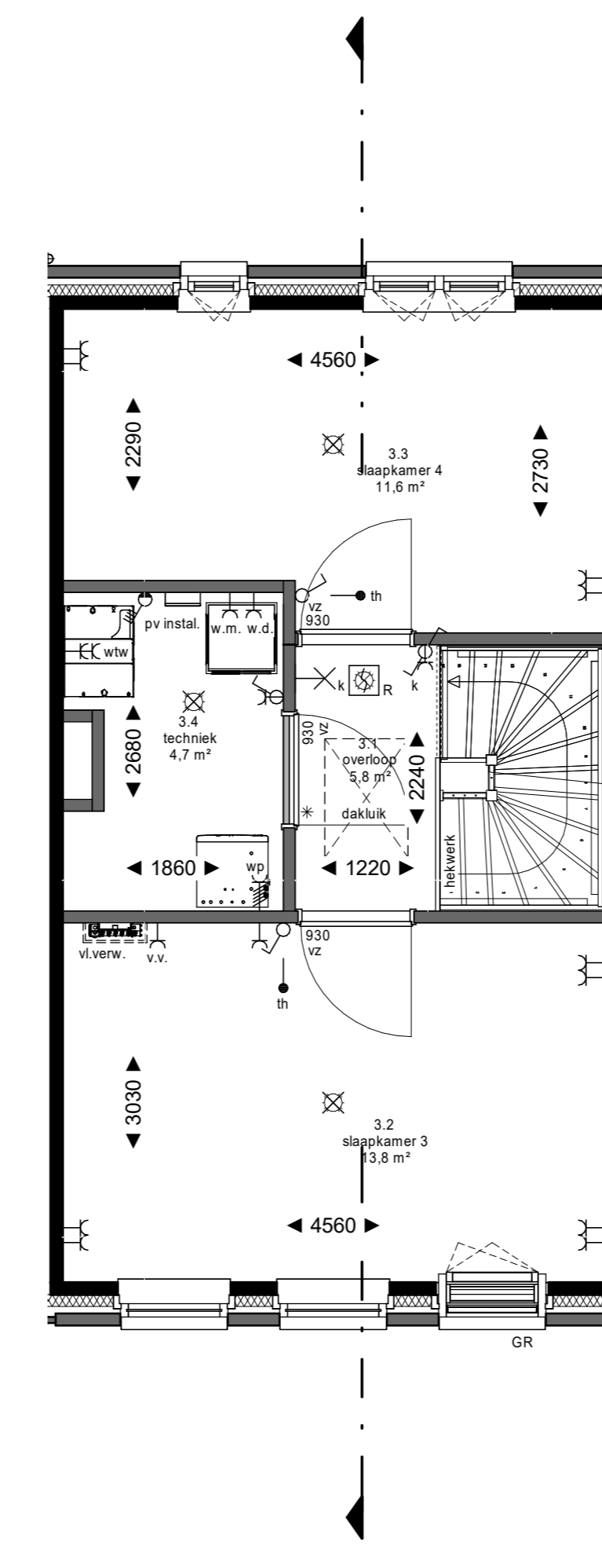
3e verdieping
