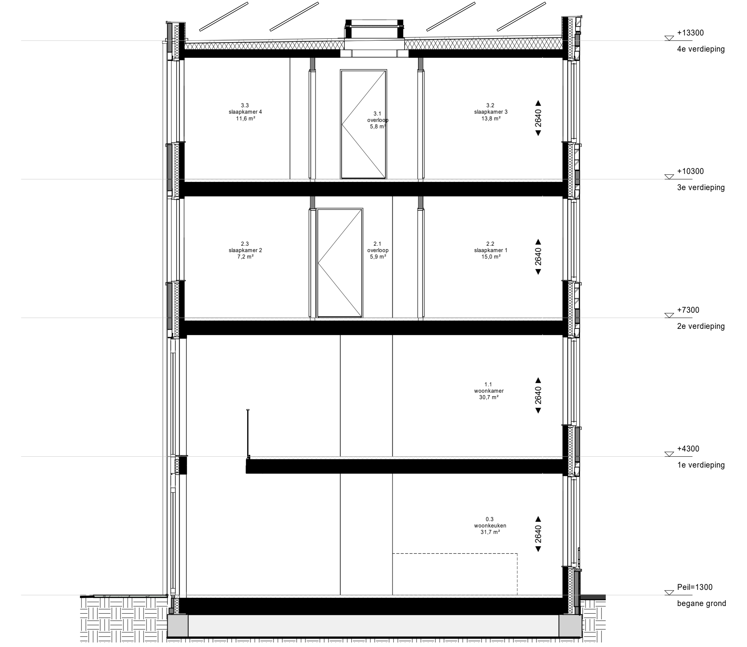
doorsnede
