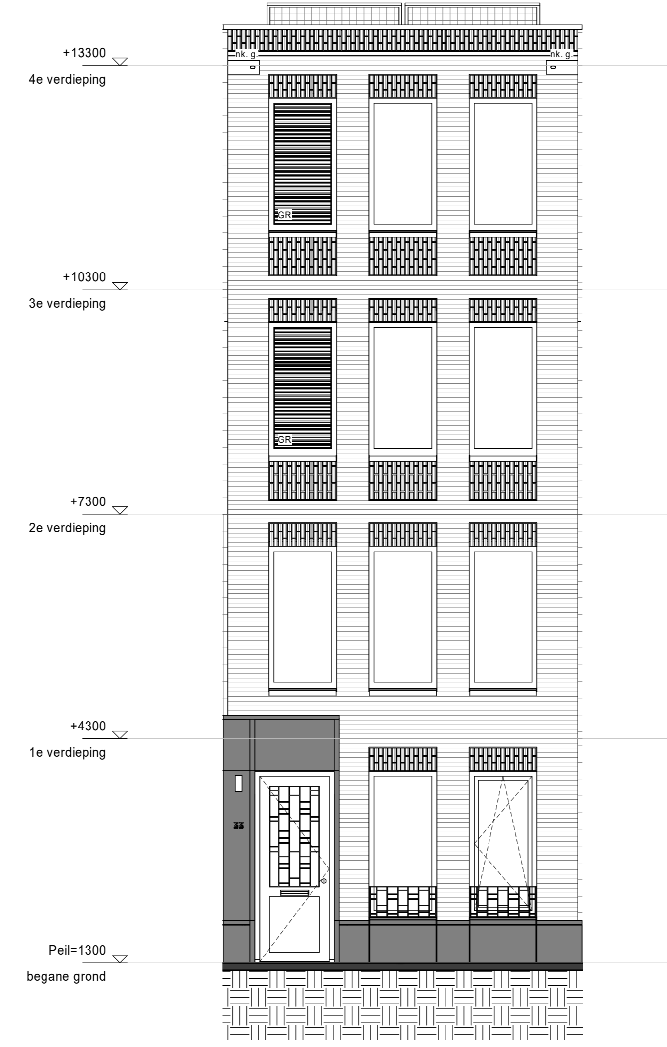
voorgevel
