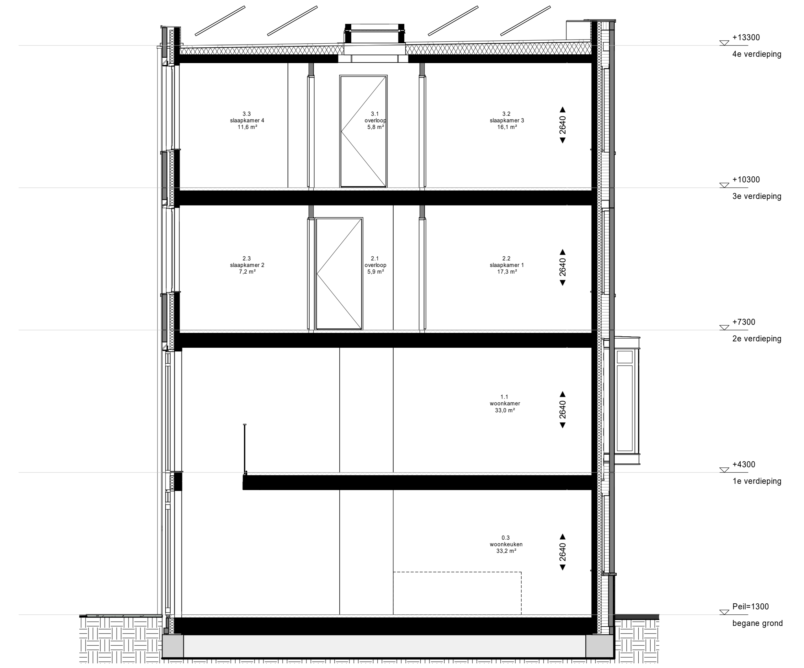
doorsnede
