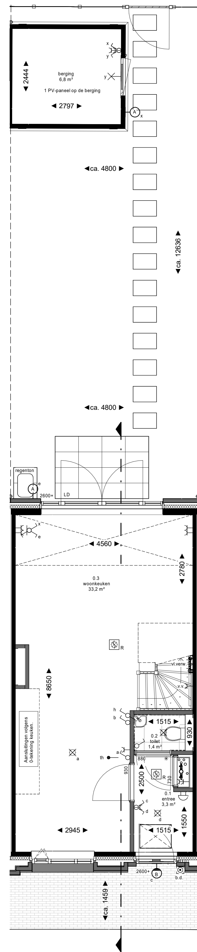
begane grond
