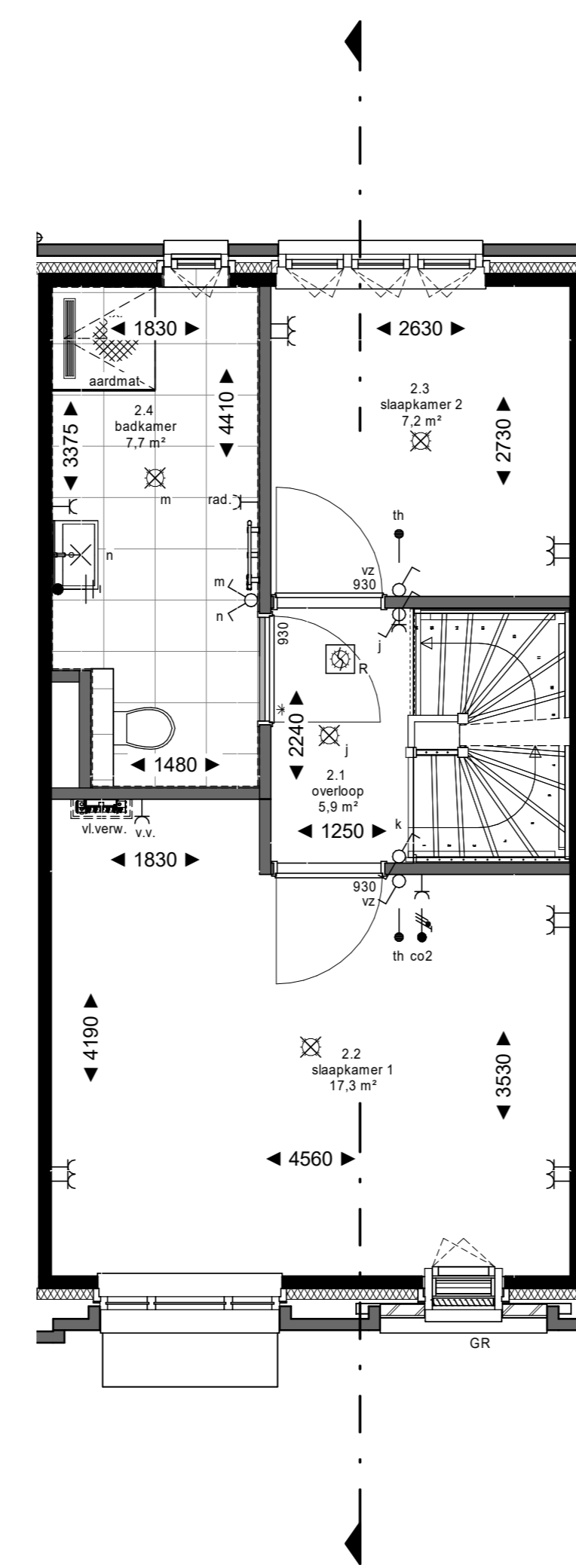
2e verdieping
