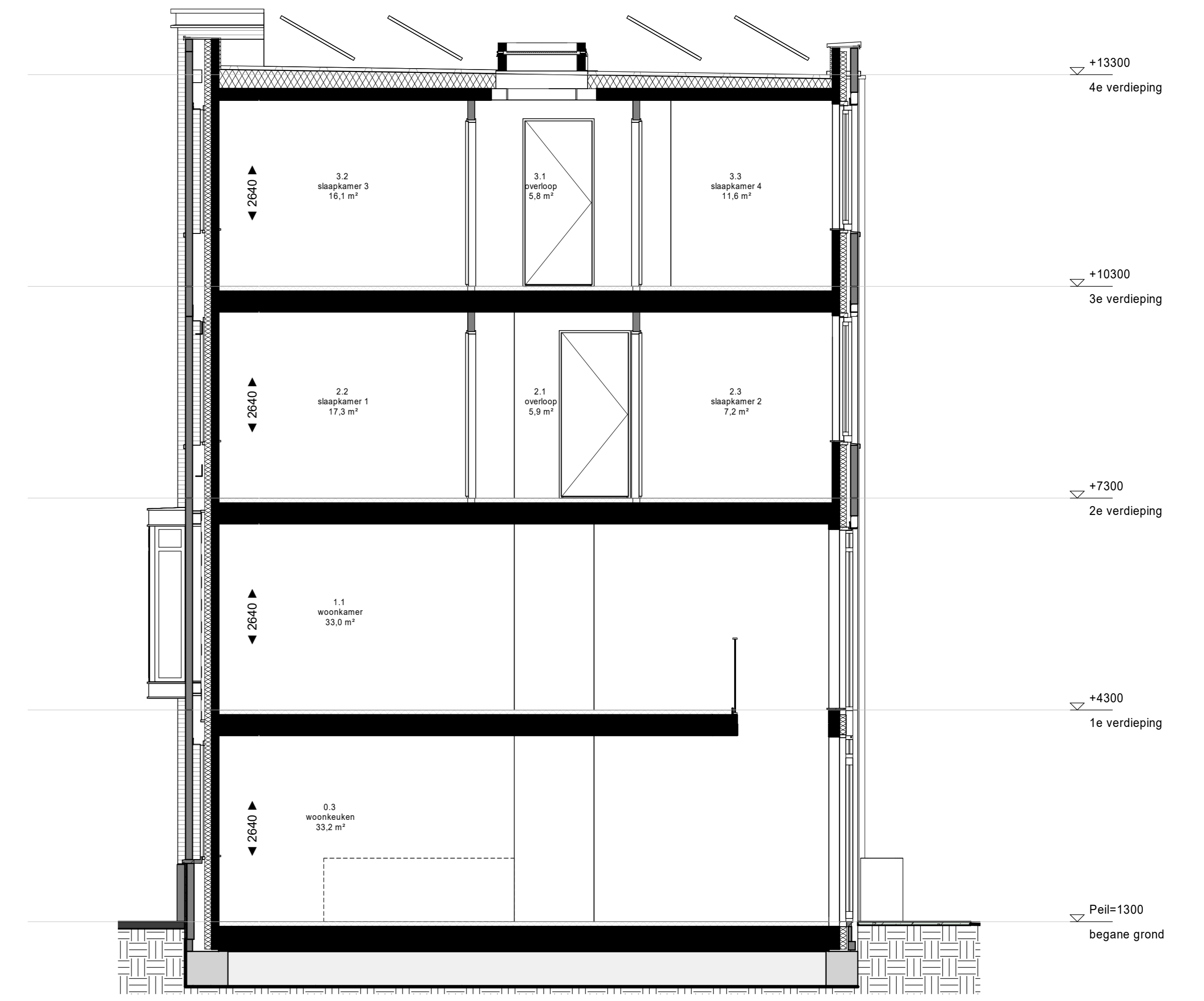
doorsnede
