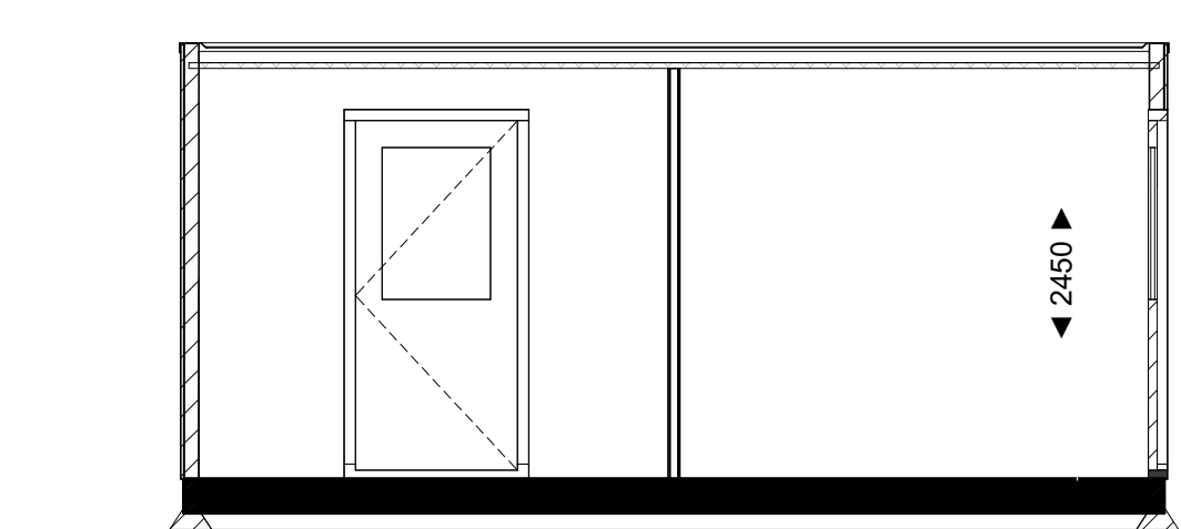
doorsnede
