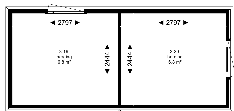
plattegrond berging 5,88m x 2,66m - gecombineerd (2 st.)
