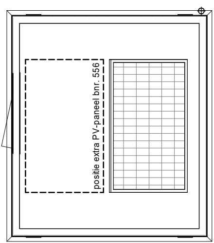
dakaanzicht
