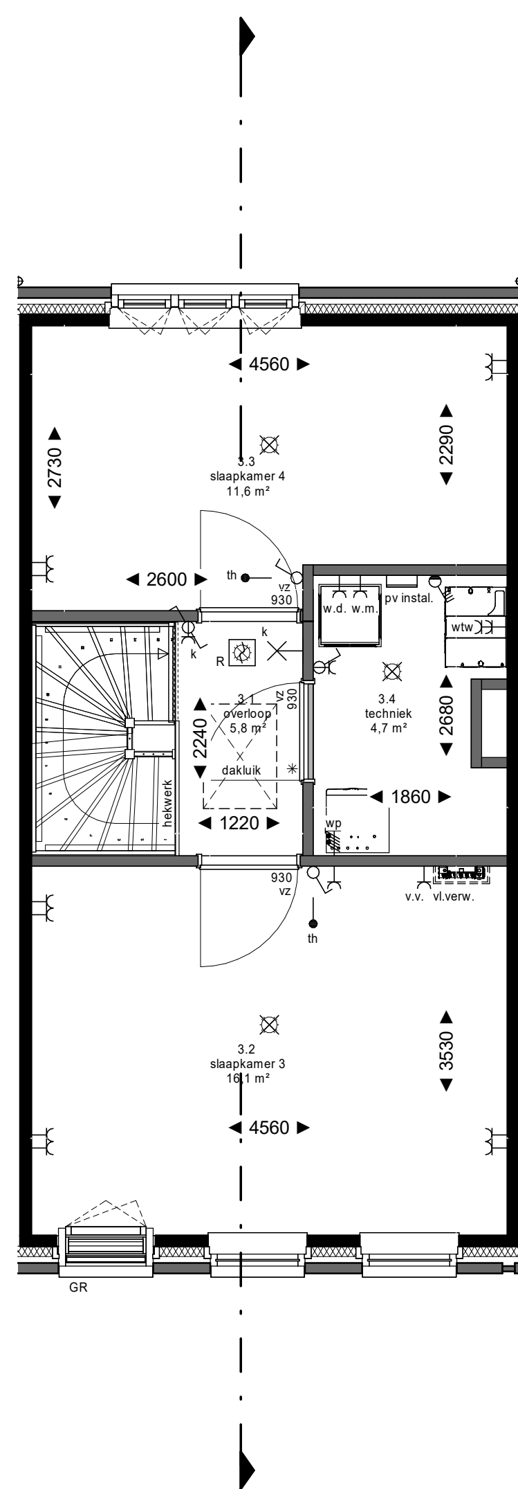
3e verdieping
