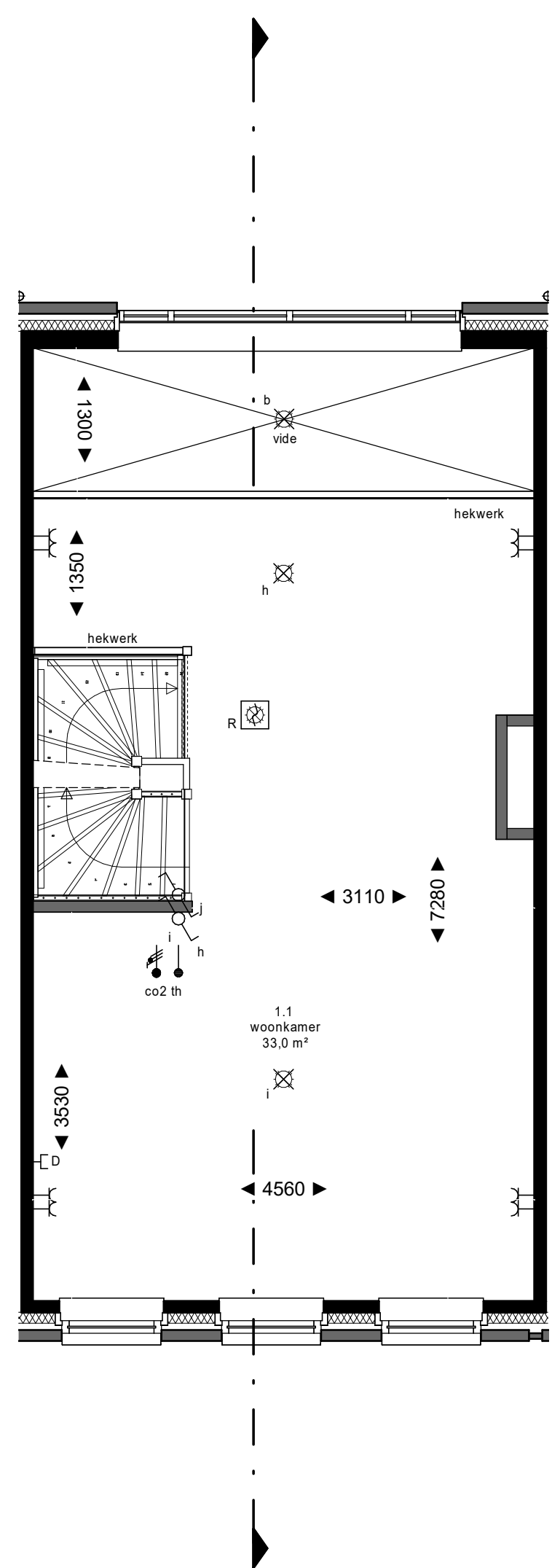
1e verdieping
