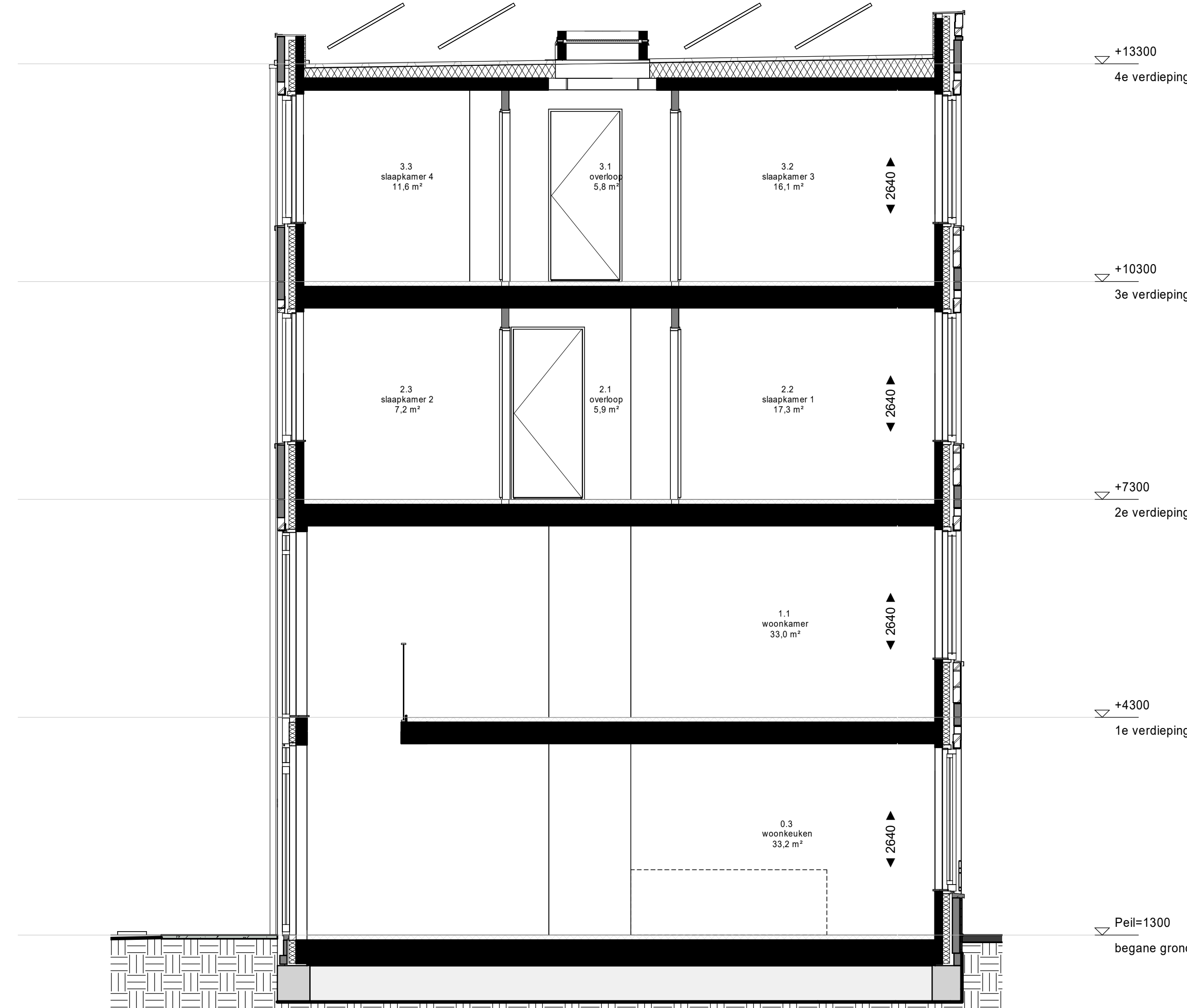
doorsnede
