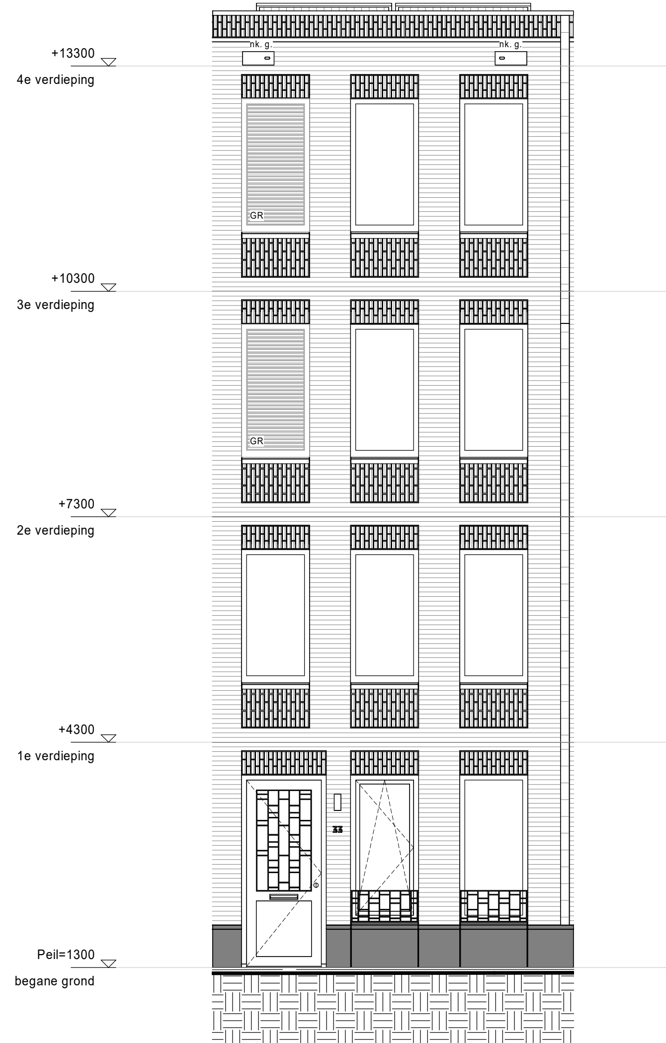
voorgevel
