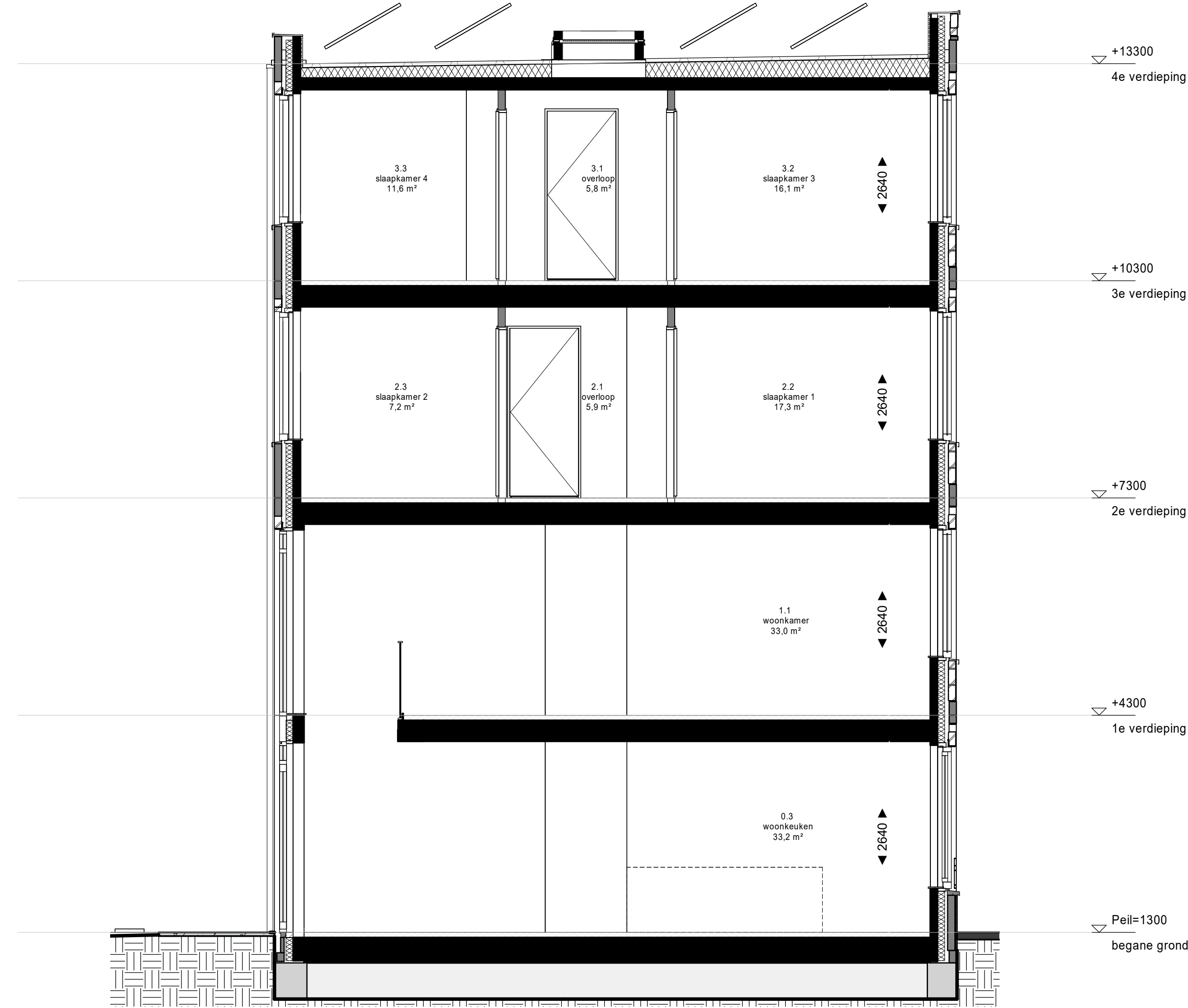
doorsnede
