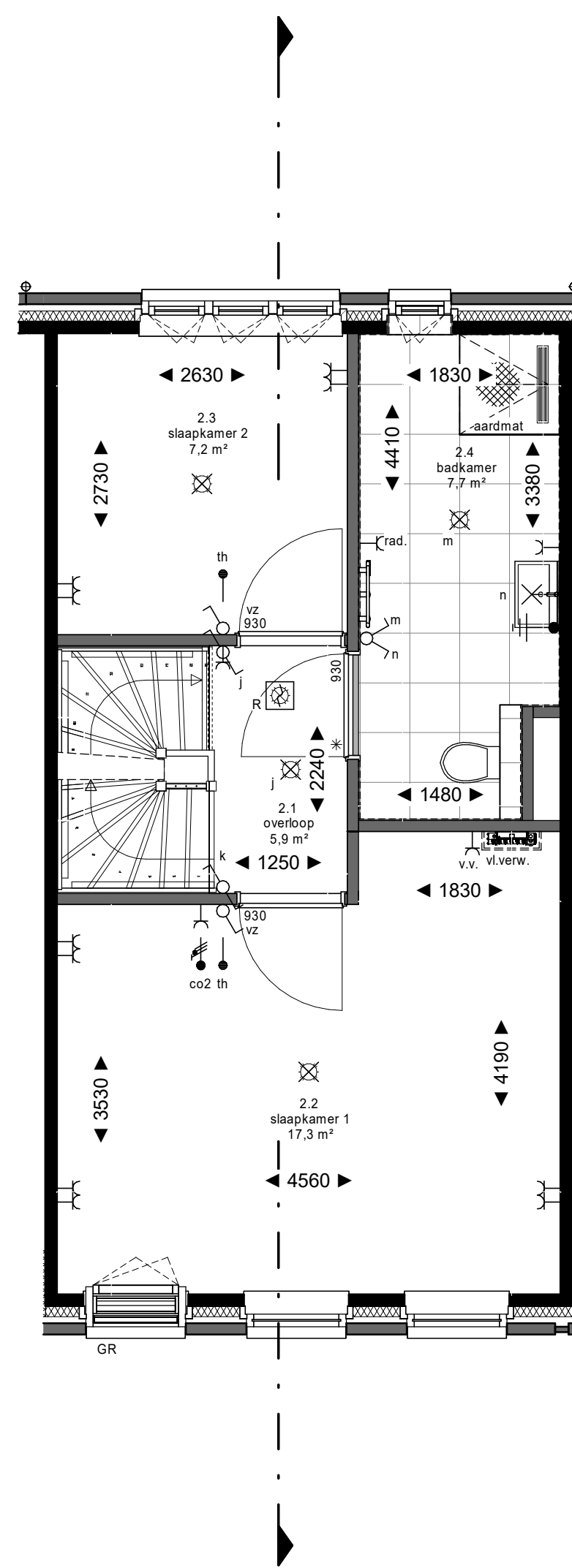
2e verdieping
