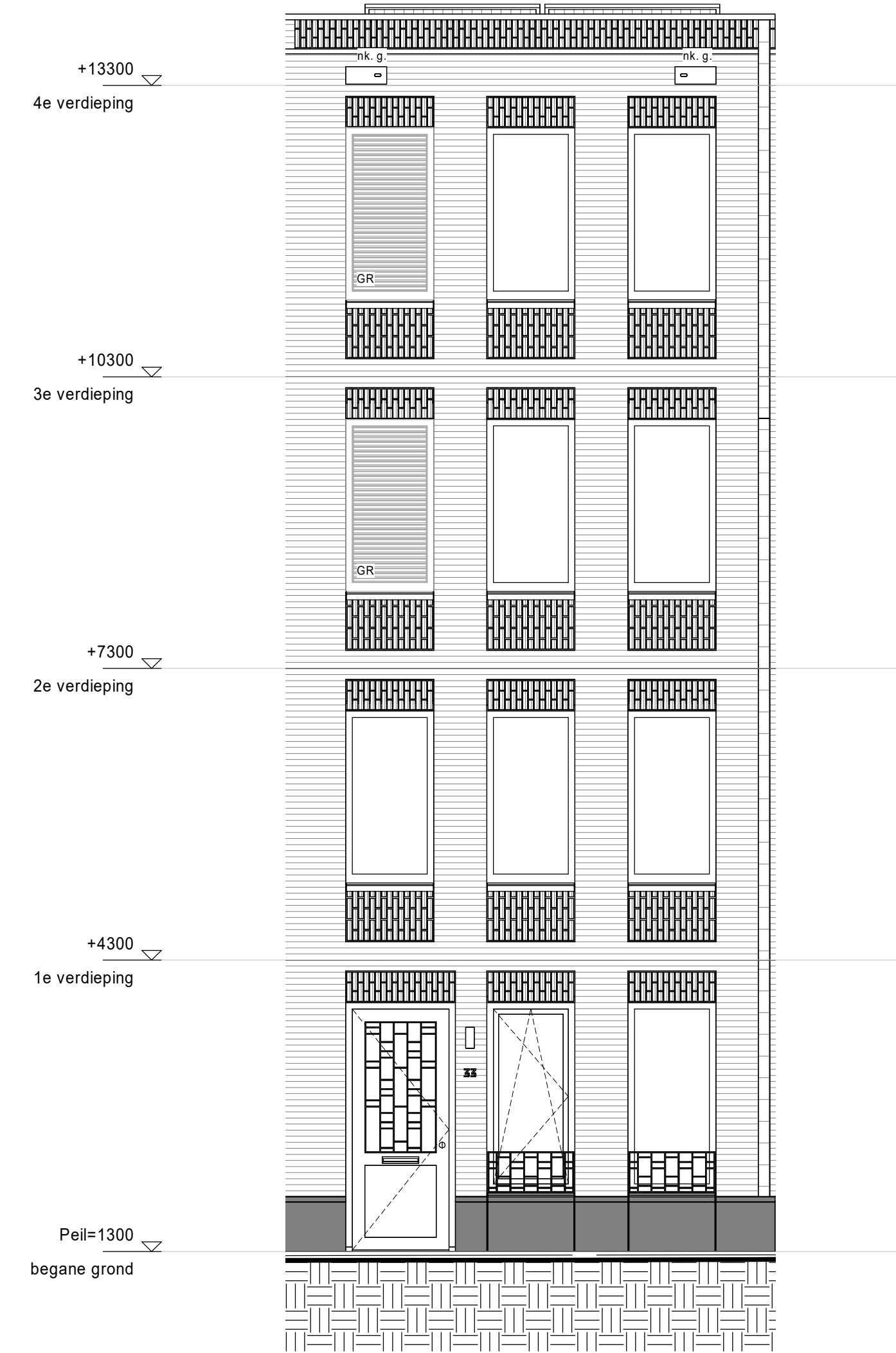
voorgevel
