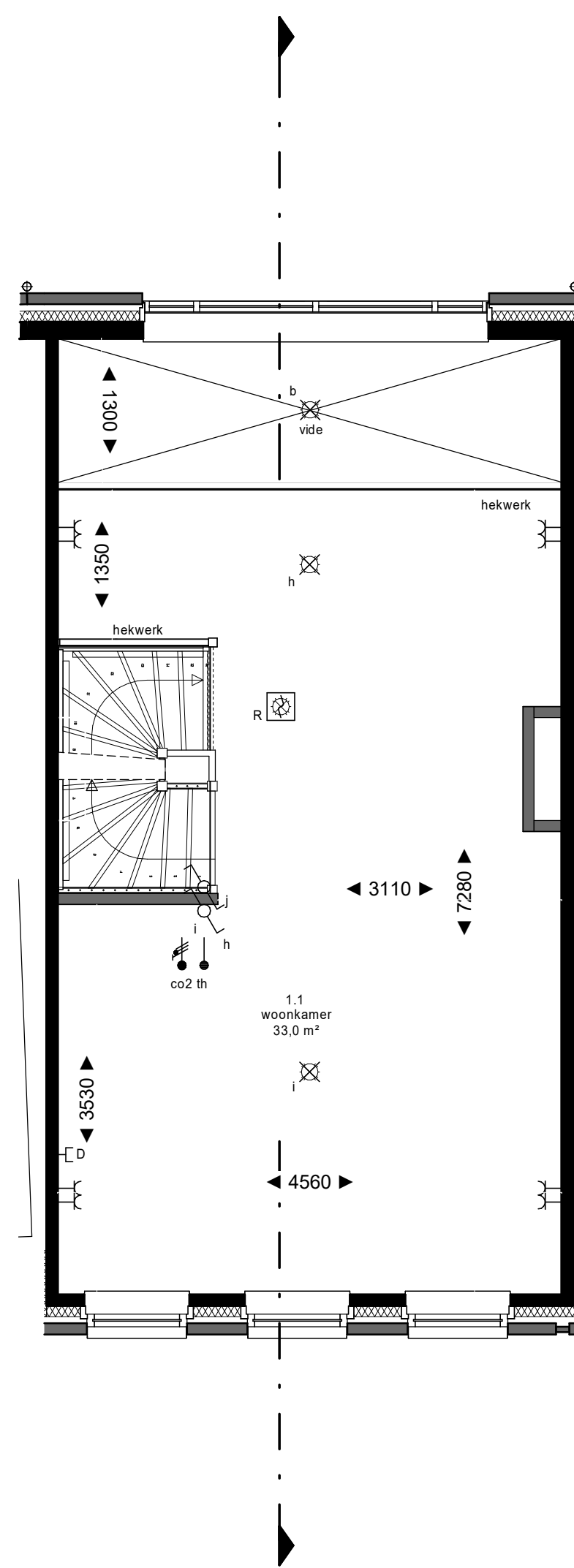
1e verdieping
