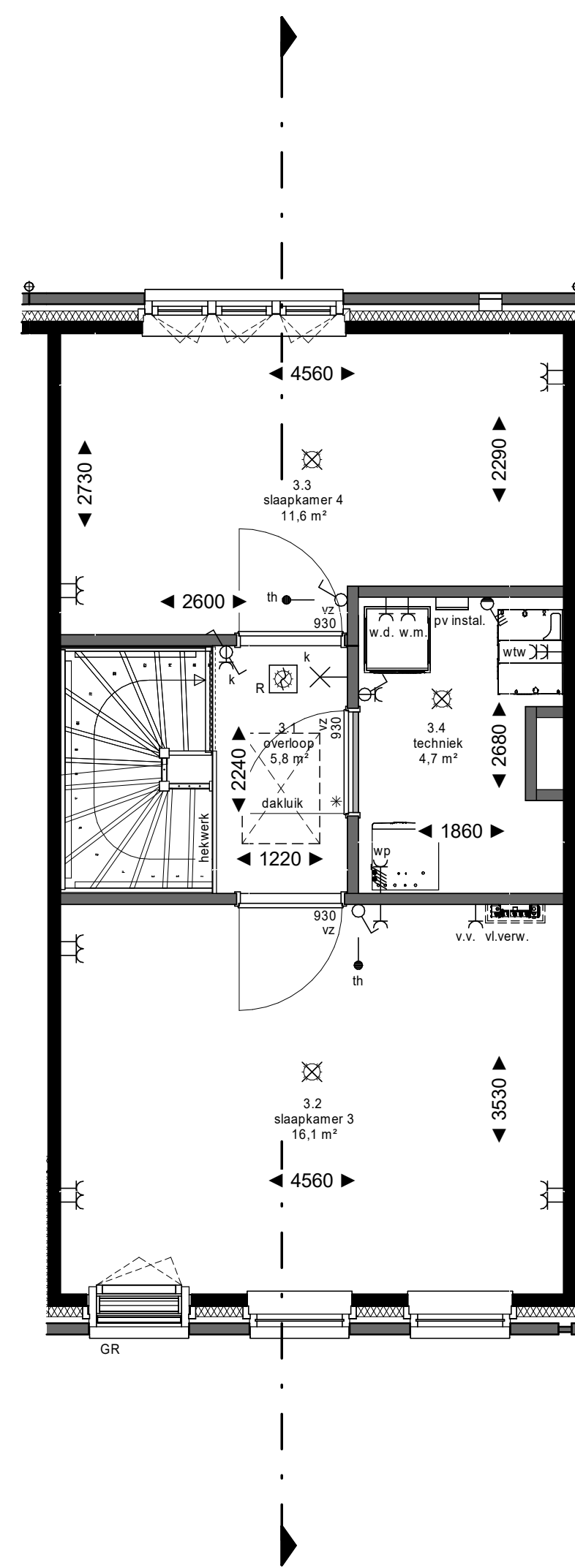
3e verdieping
