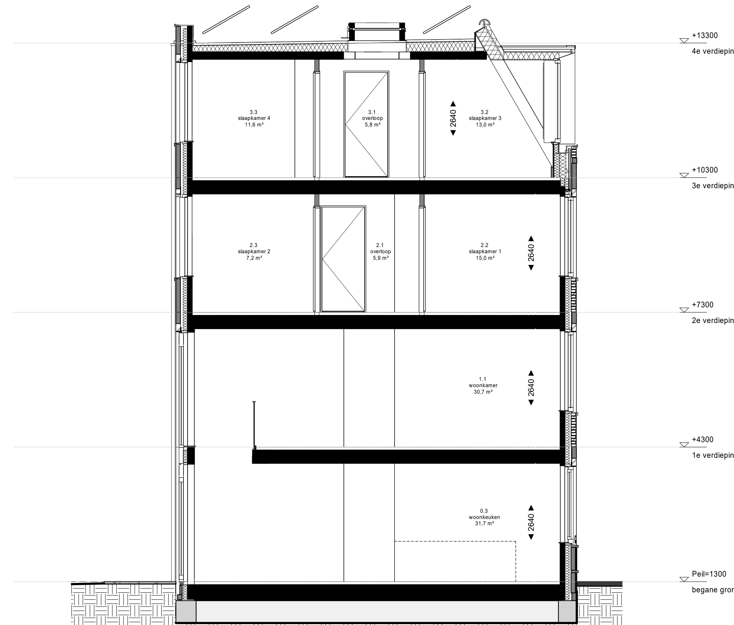
doorsnede
