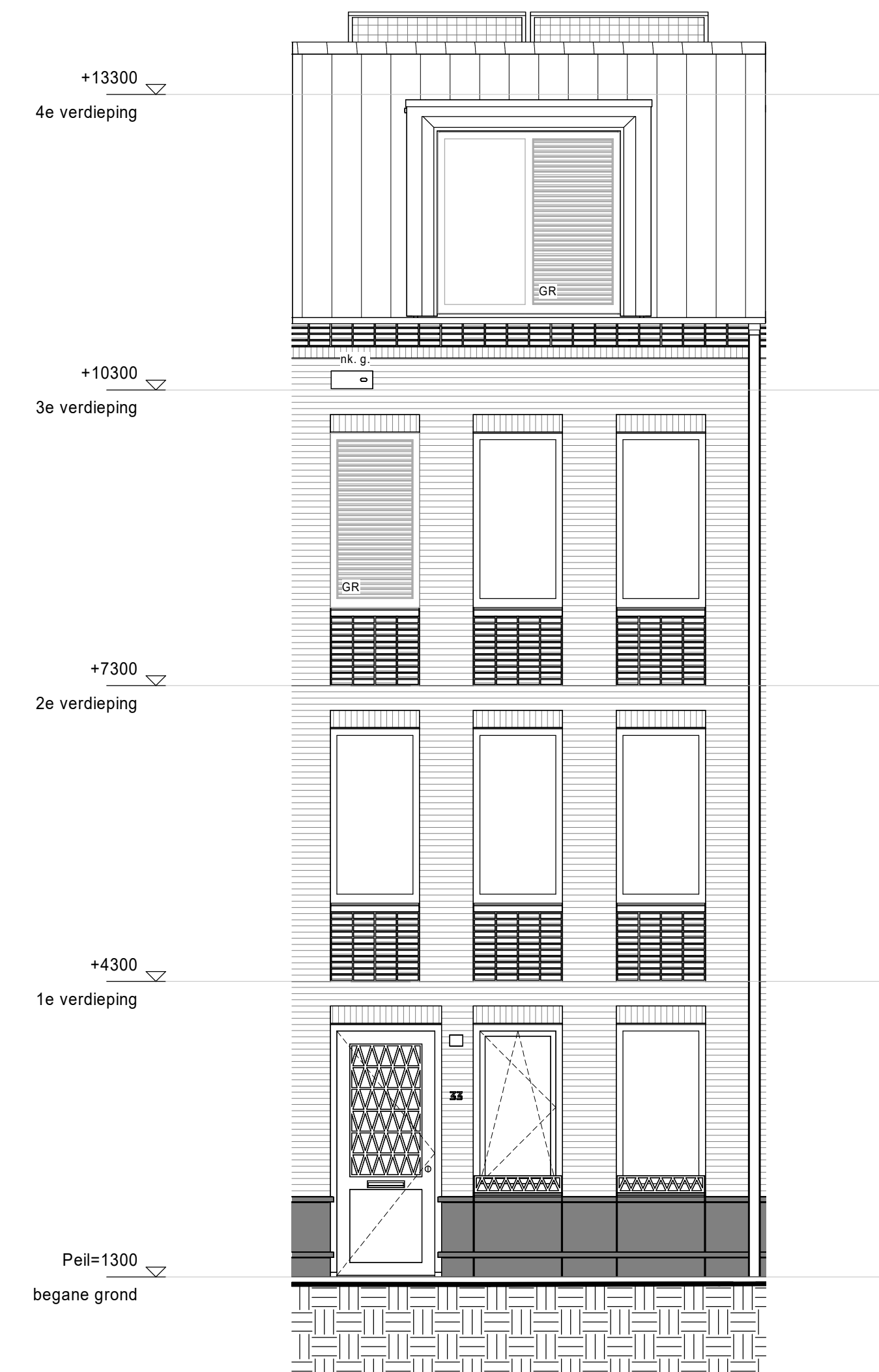
voorgevel
