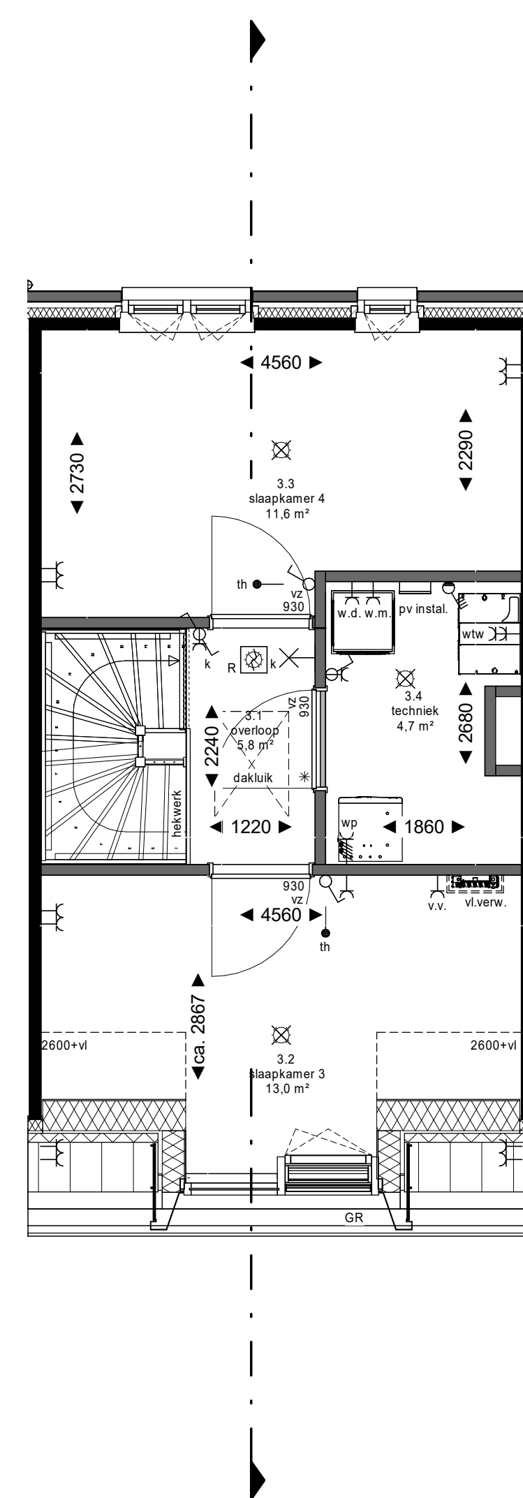
3e verdieping
