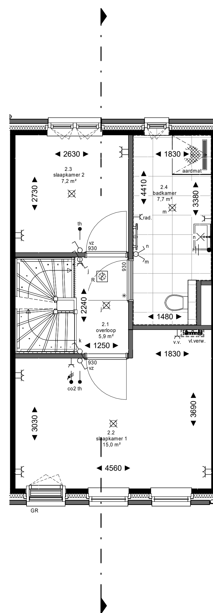
2e verdieping
