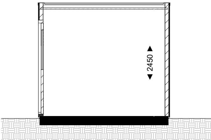
doorsnede
