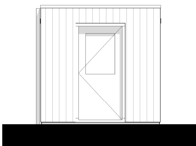
voorgevel
