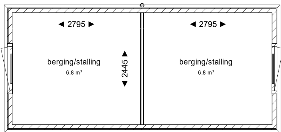
plattegrond berging 5,88m x 2,66m - gecombineerd (14 stuks)
