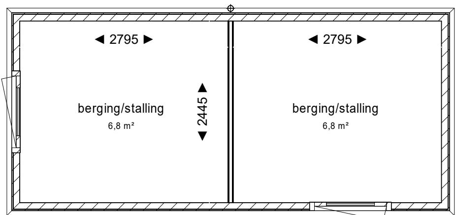
plattegrond berging 5,88m x 2,66m - gecombineerd (3 stuks, waarvan 1 getekend en 2 gespiegeld)
