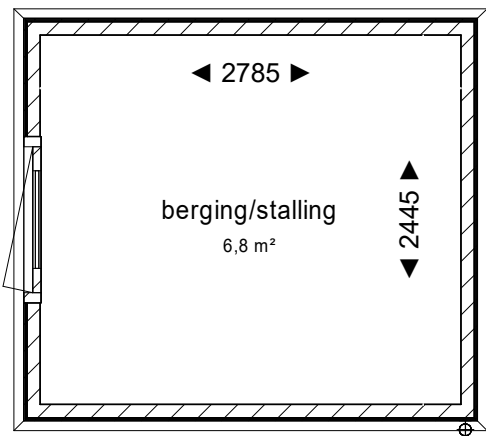
plattegrond berging 3m x 2,66m - vrijstaand (4 stuks, waarvan 1 getekend en 3 gespiegeld)
