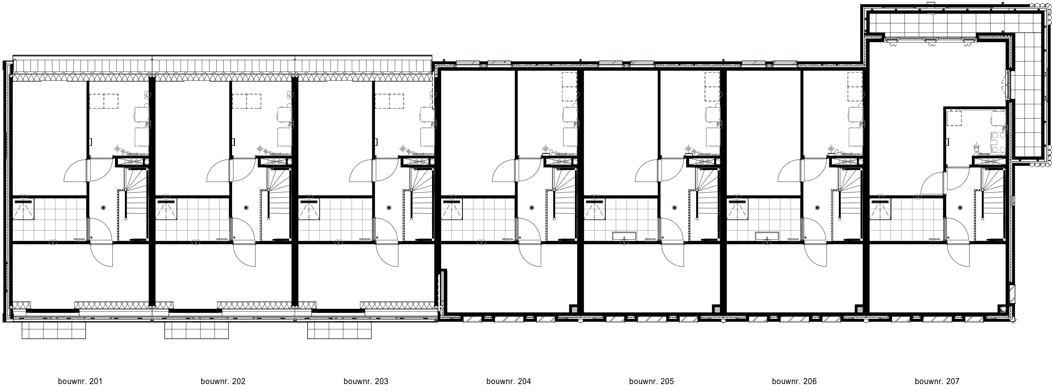
2e verdieping
