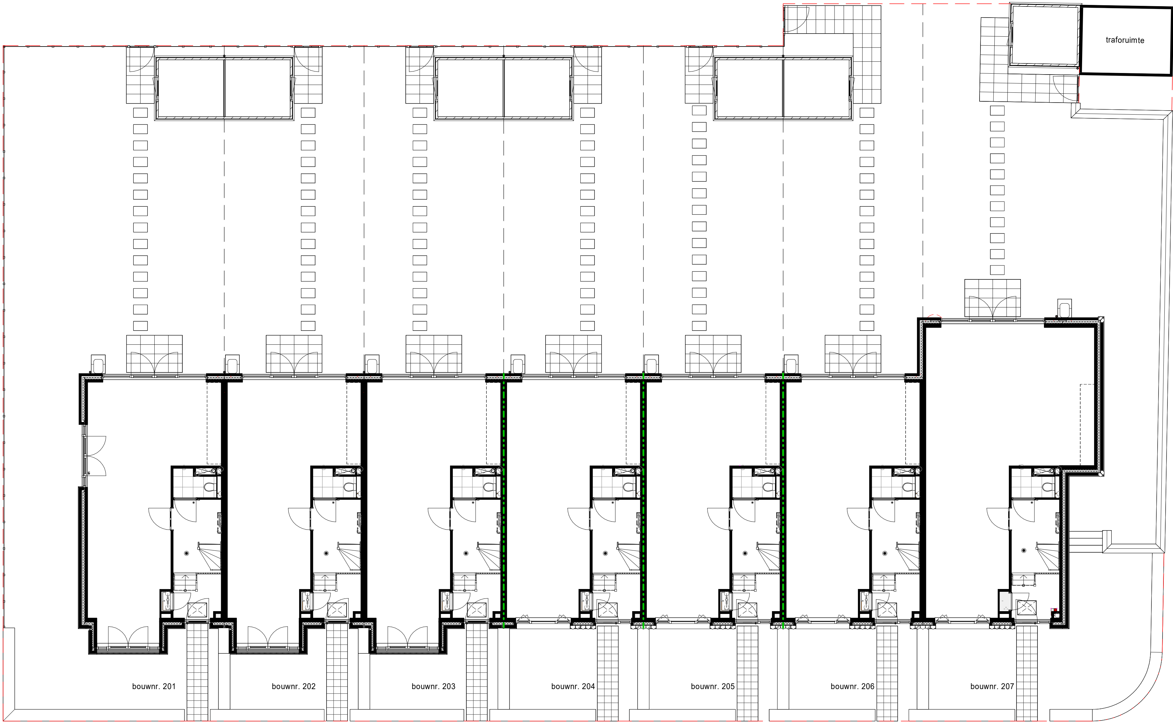
begane grond
