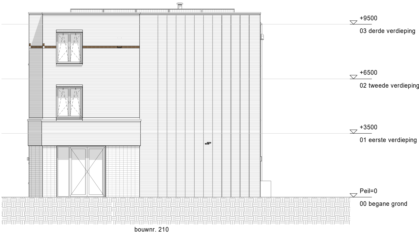
rechtergevel
