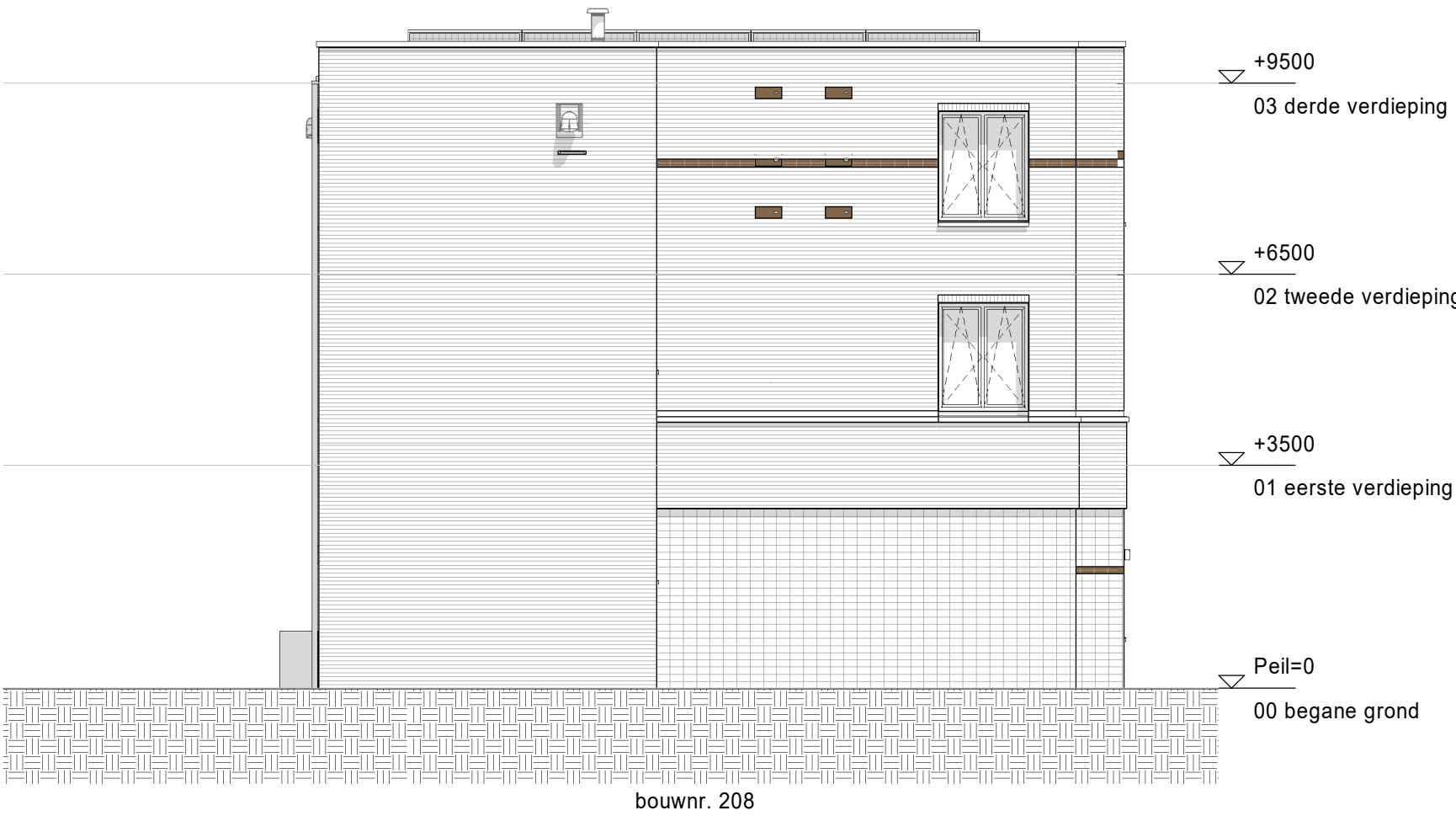
linkergevel
