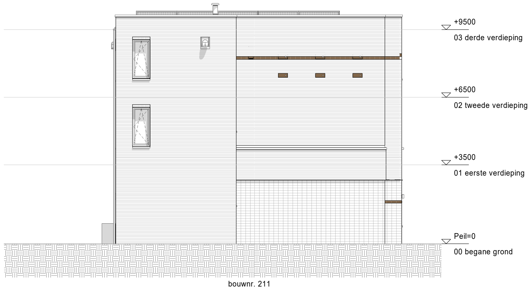
linkergevel
