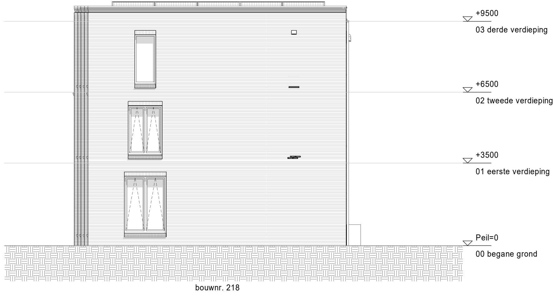
rechtergevel
