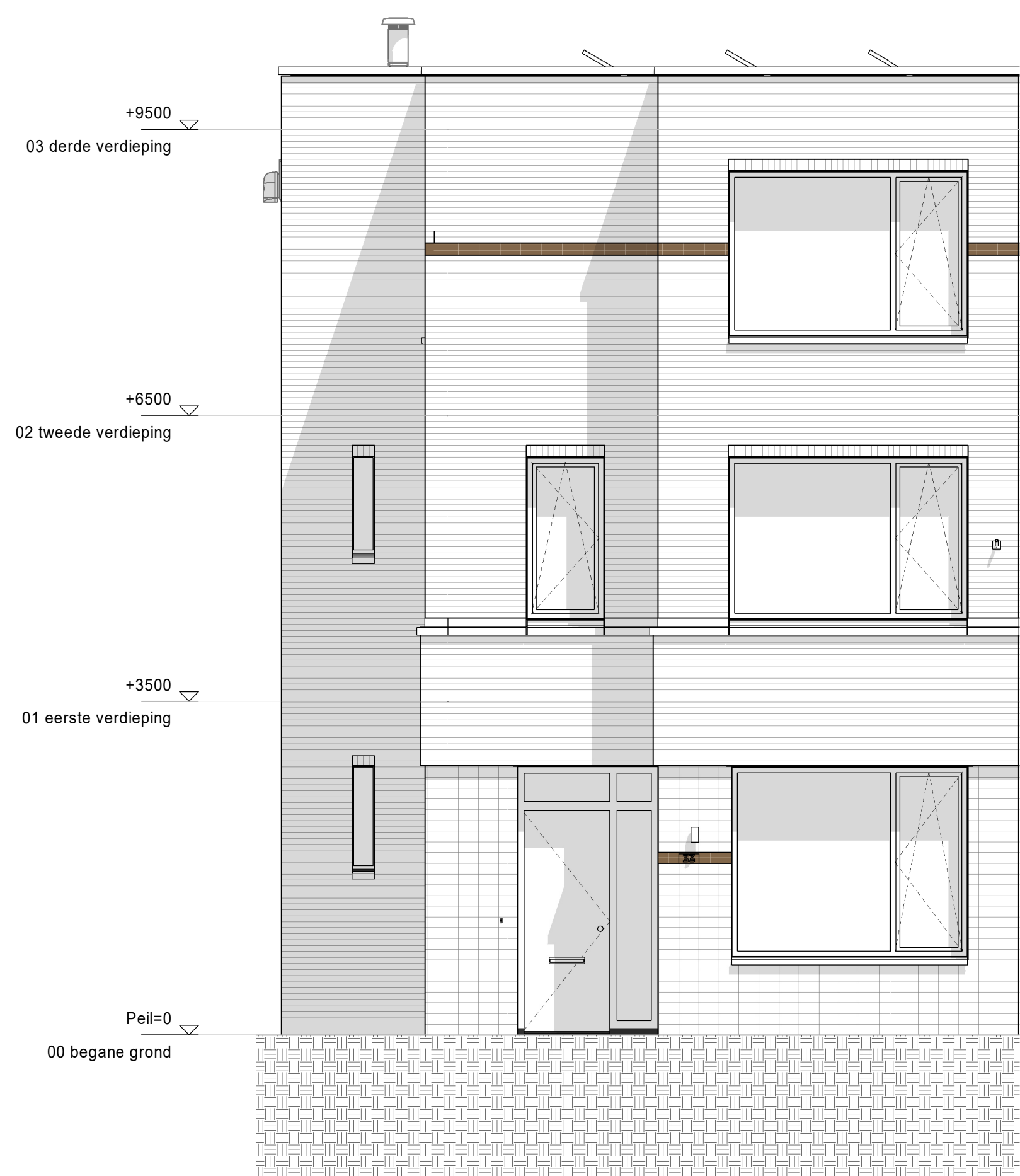
voorgevel
