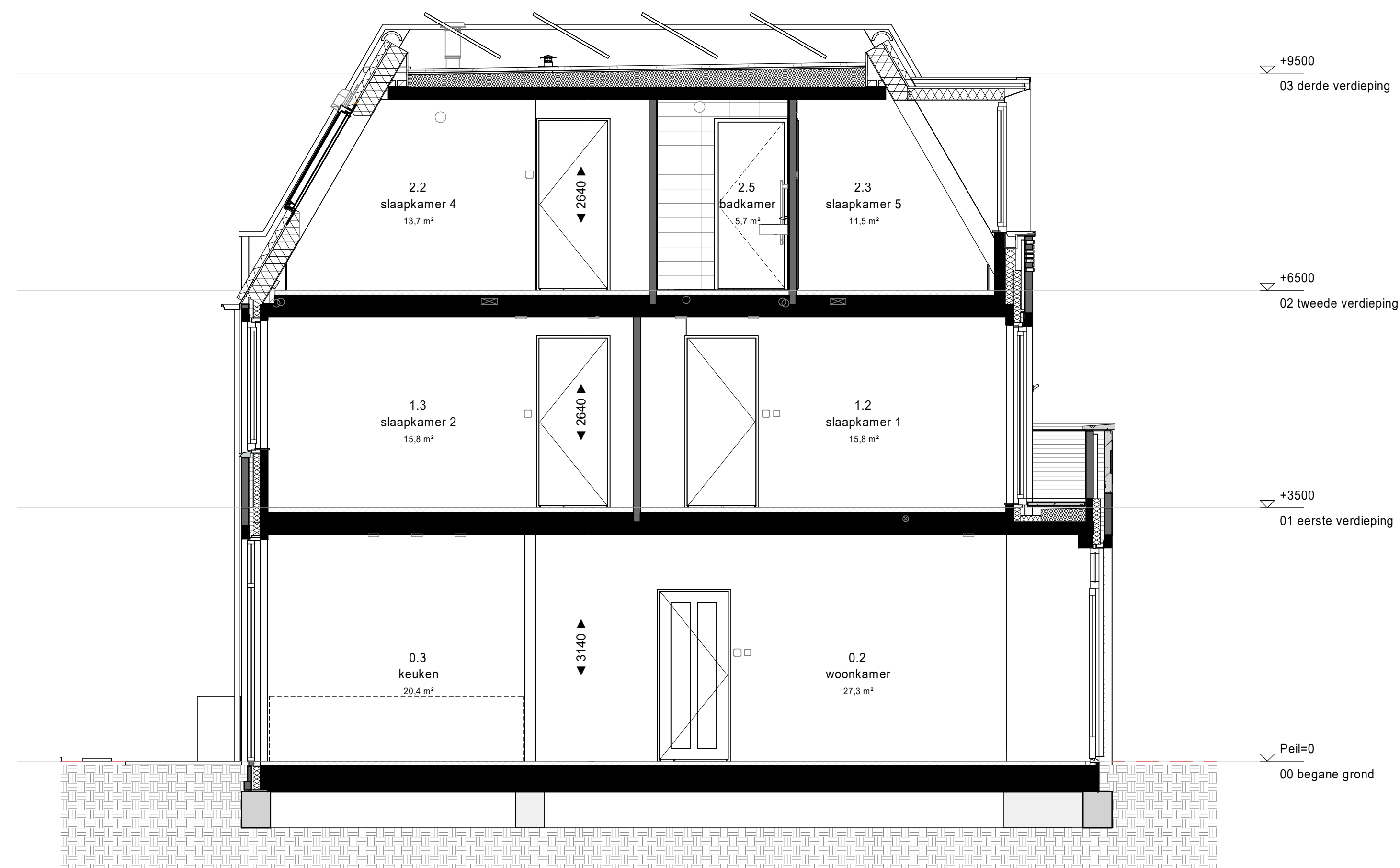
doorsnede
