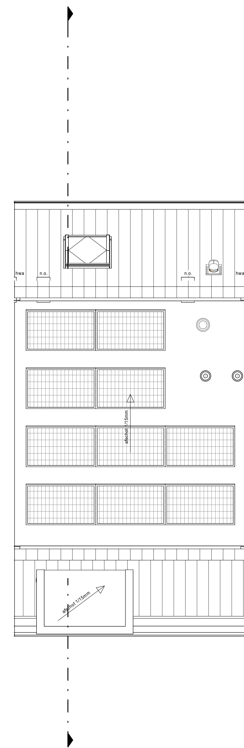
dakoverzicht
