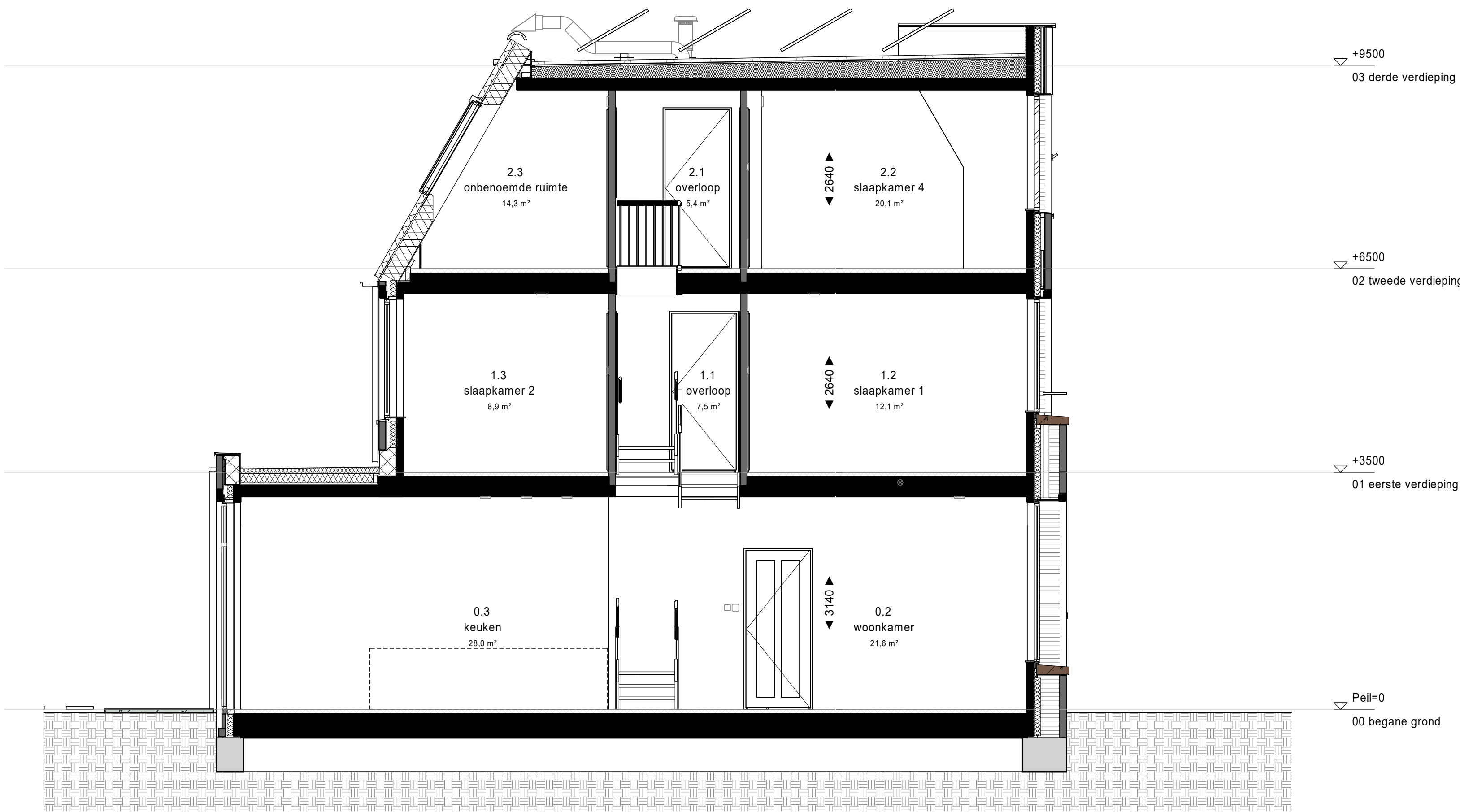
doorsnede
